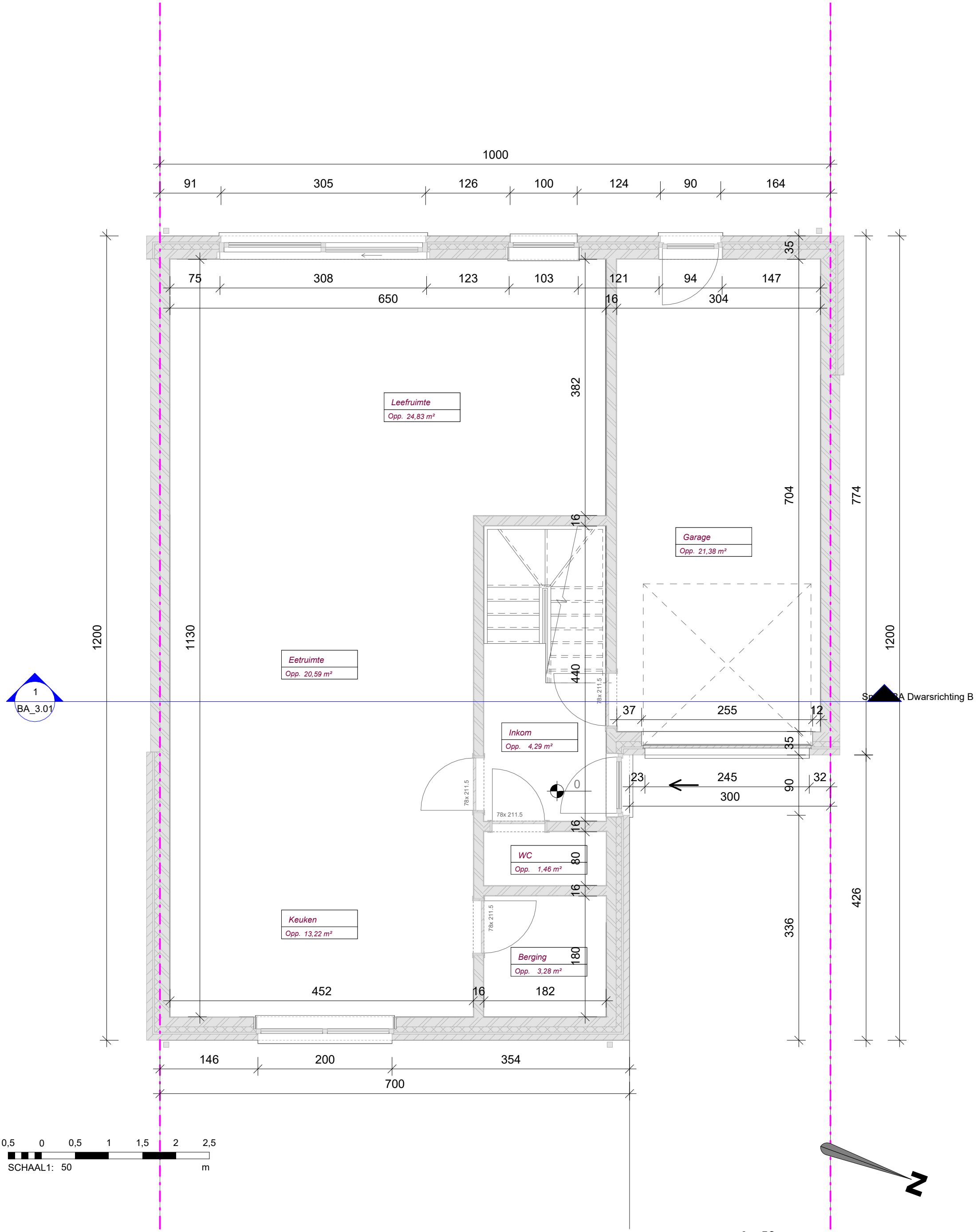
BA_1.00 P_B_1.00_Grondplan Gelijkvloers
