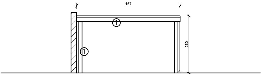
Voorgevel 1/100
