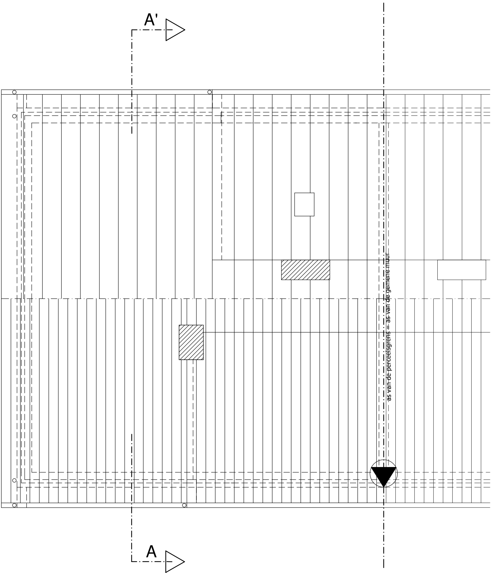
DAKENPLAN bestaande toestand dakoppervlak 69,4 m 2 schaal 1/50
