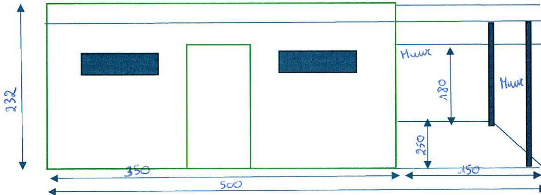
Voorzijaanzicht
