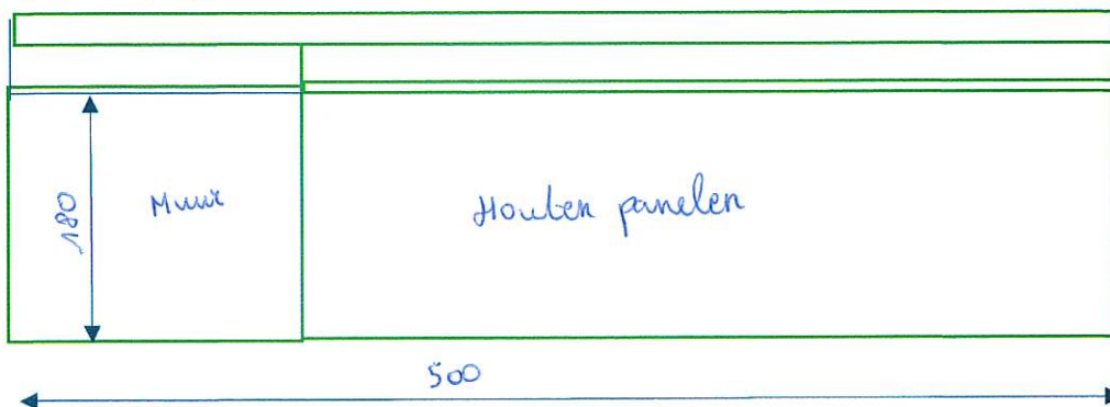
Achterzijaanzicht
