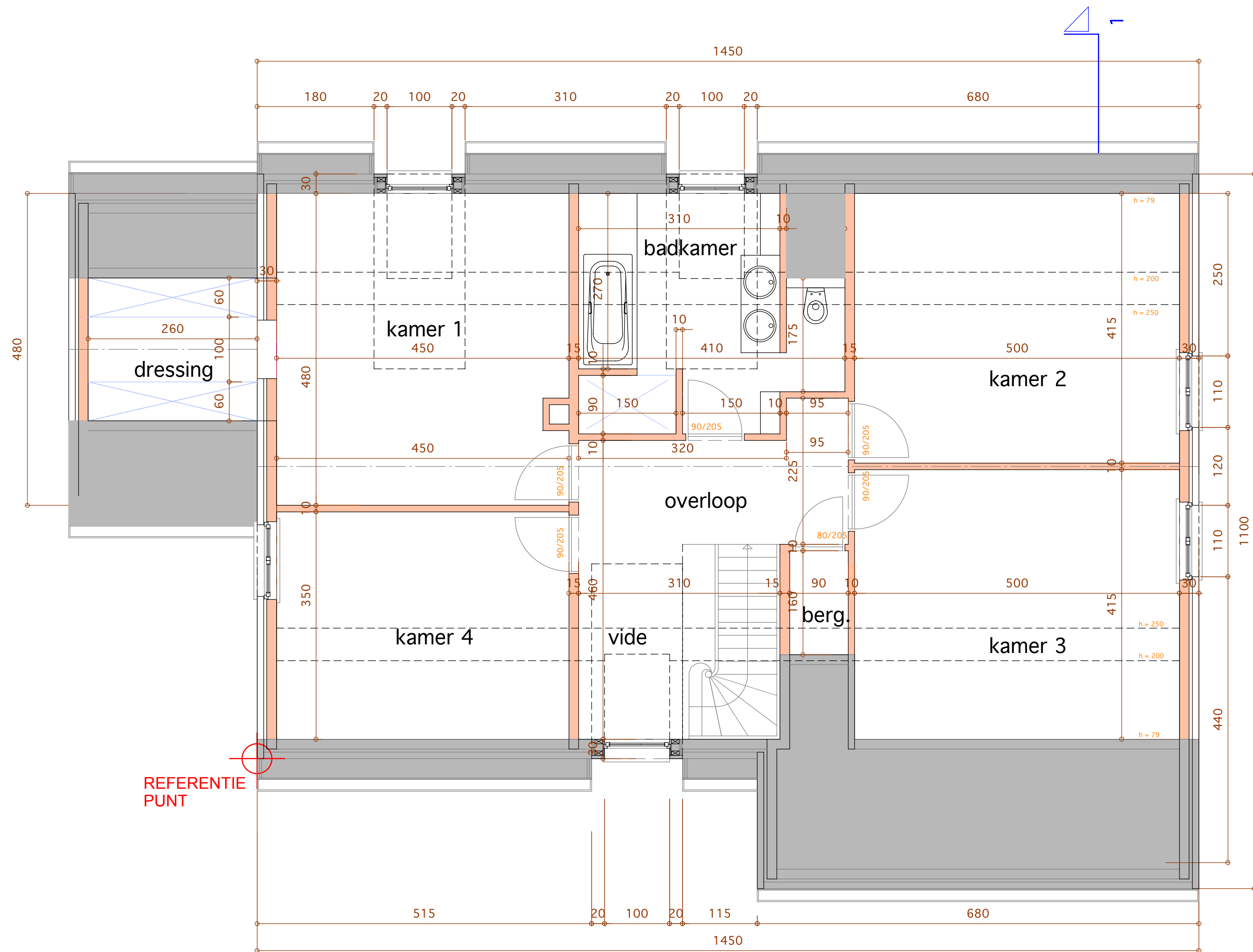
verdiepingsplan bestaande toestand
