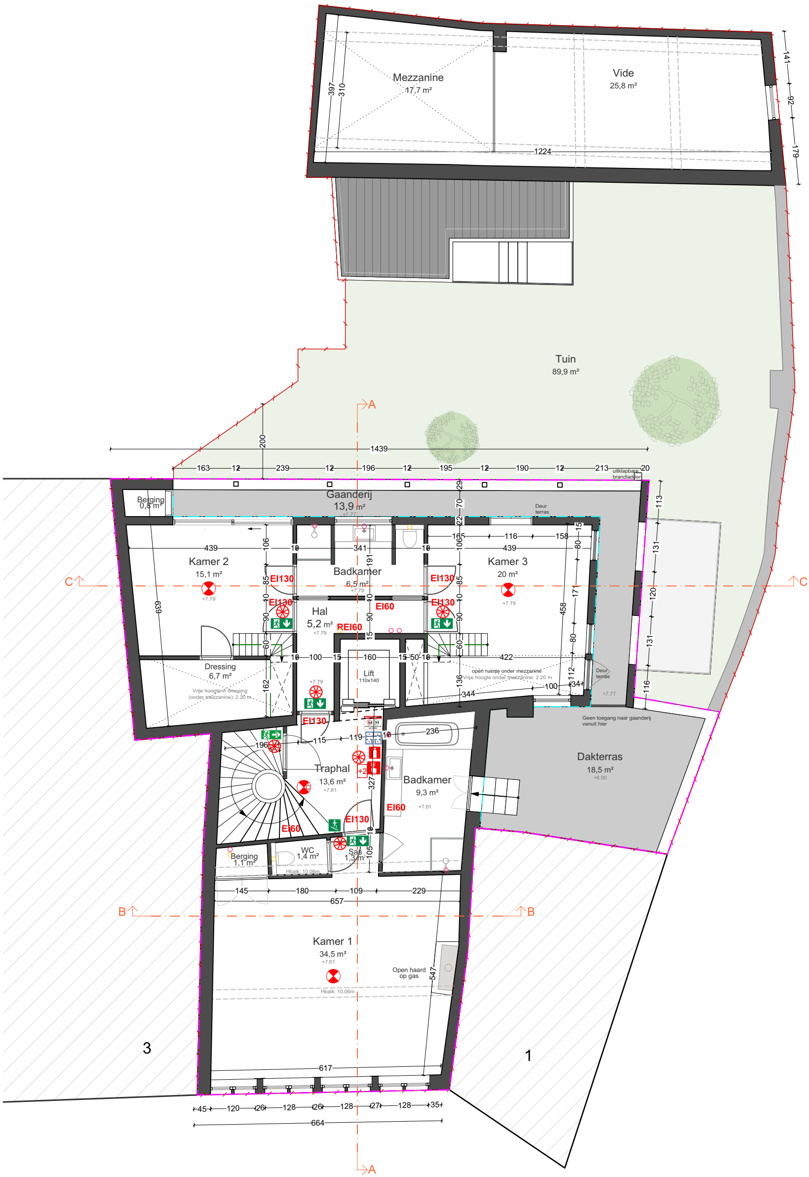
Korenlei nr 2 TWEDE VERDIEPING BVowonen = 0
