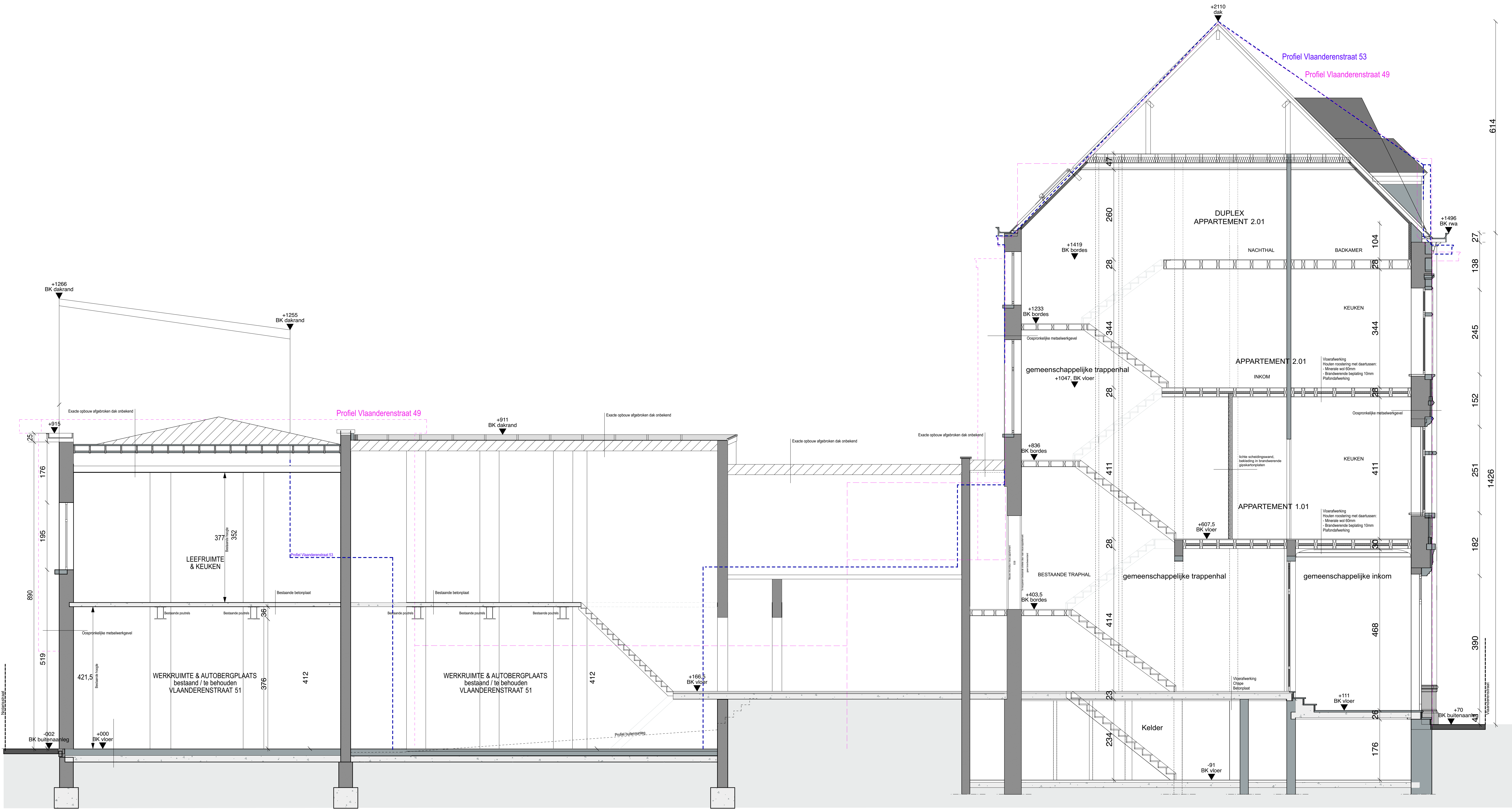
Doorsnede BB, vergunde toestand Schaal: 1/50
