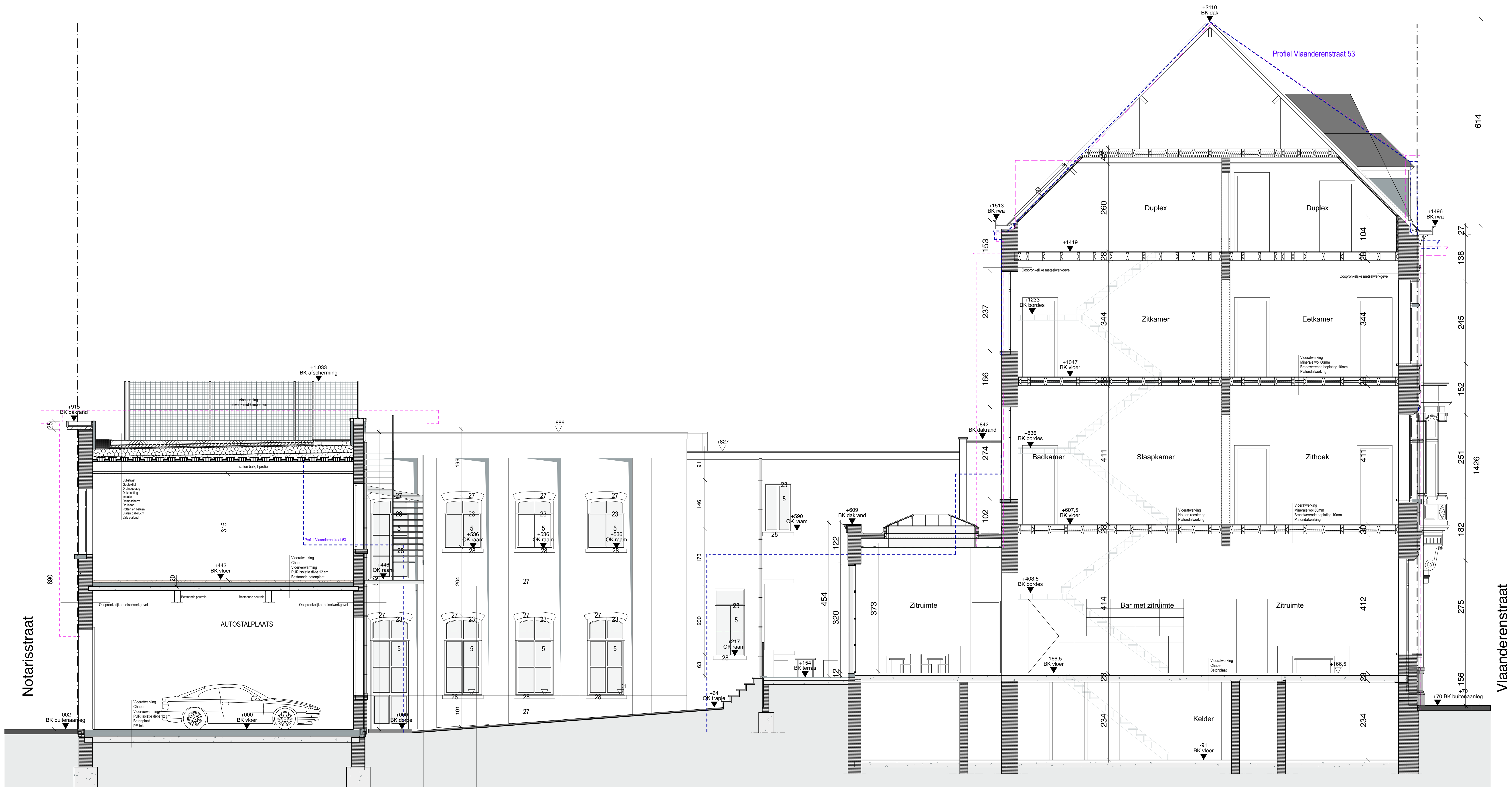
Doorsnede AA, bestaande toestand Schaal: 1/50
