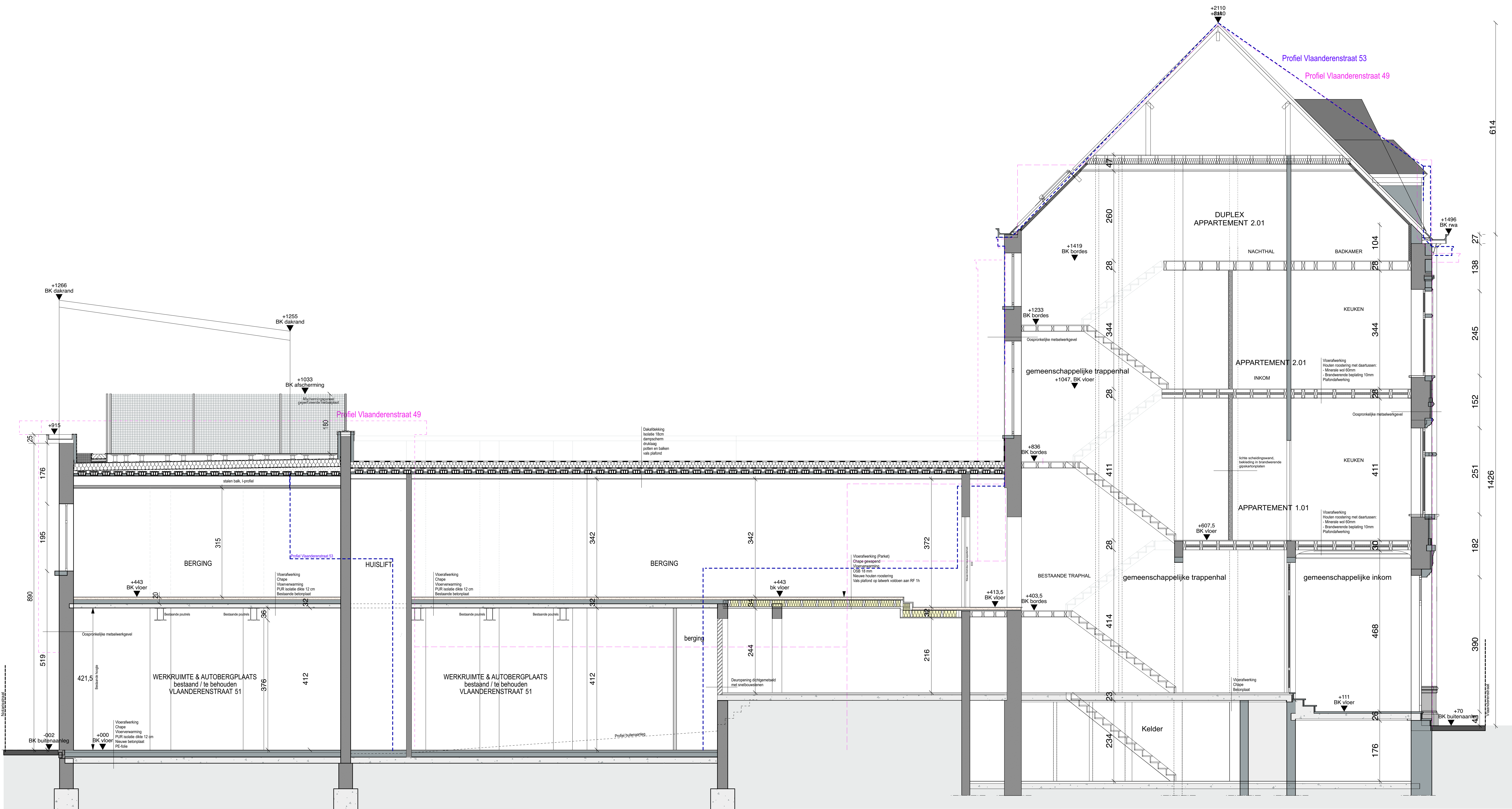
Doorsnede BB, bestaande toestand Schaal: 1/50
