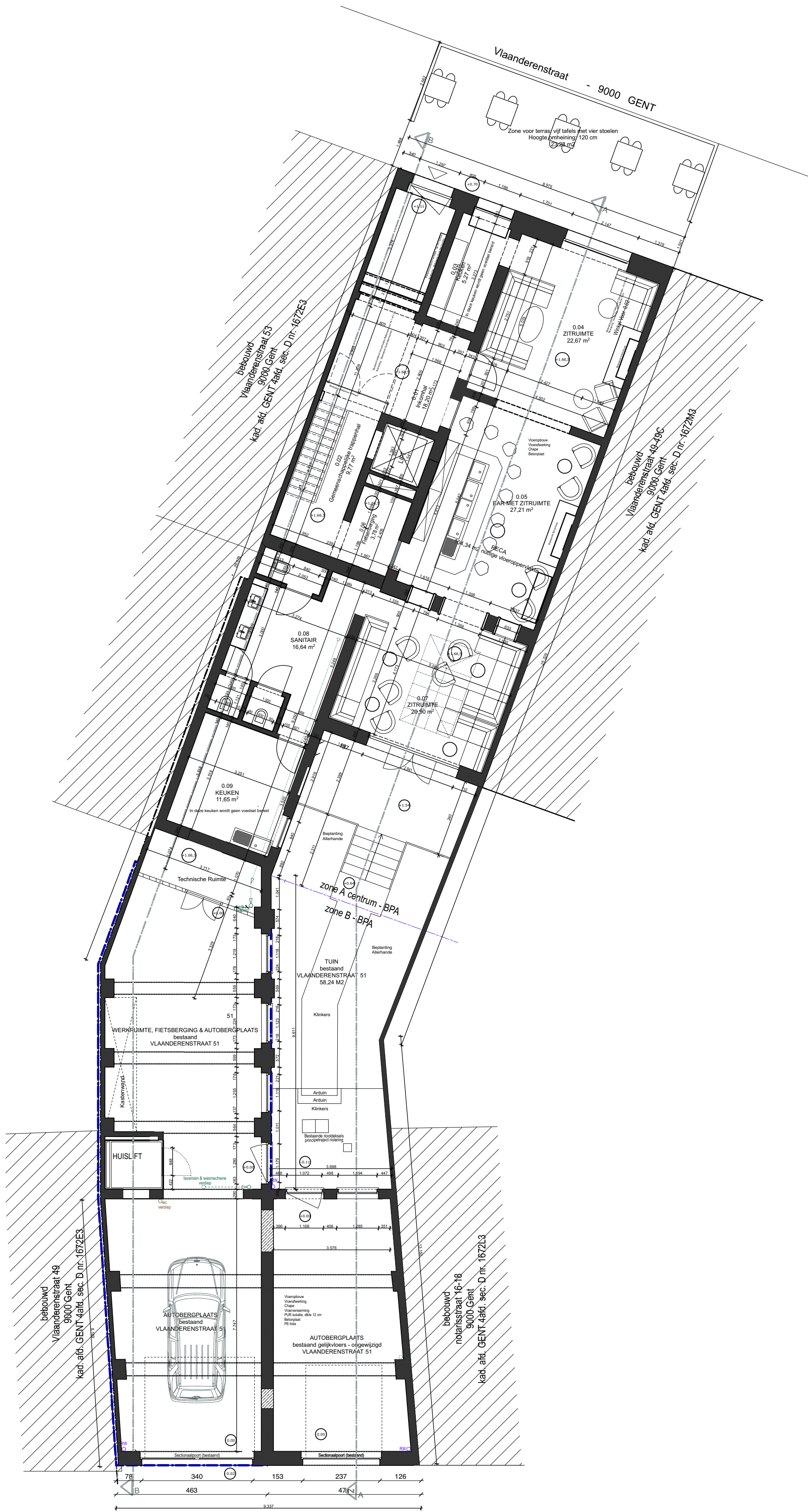
Geijkvloerse verdieping, bestaande toestand Schaal: 1/50
