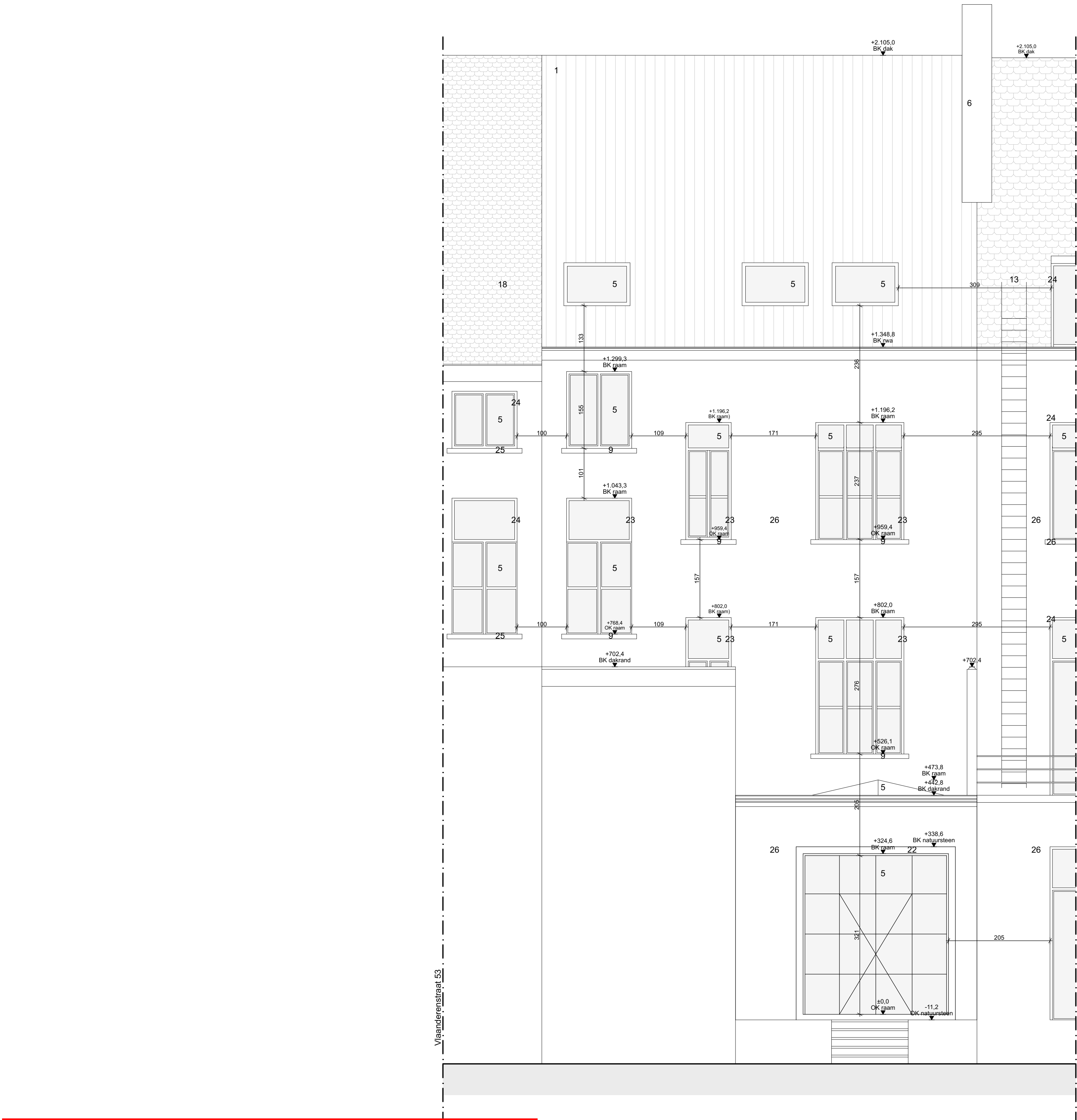
Achtergevel hoofdgebouw, nieuwe toestand Schaal 1/50
