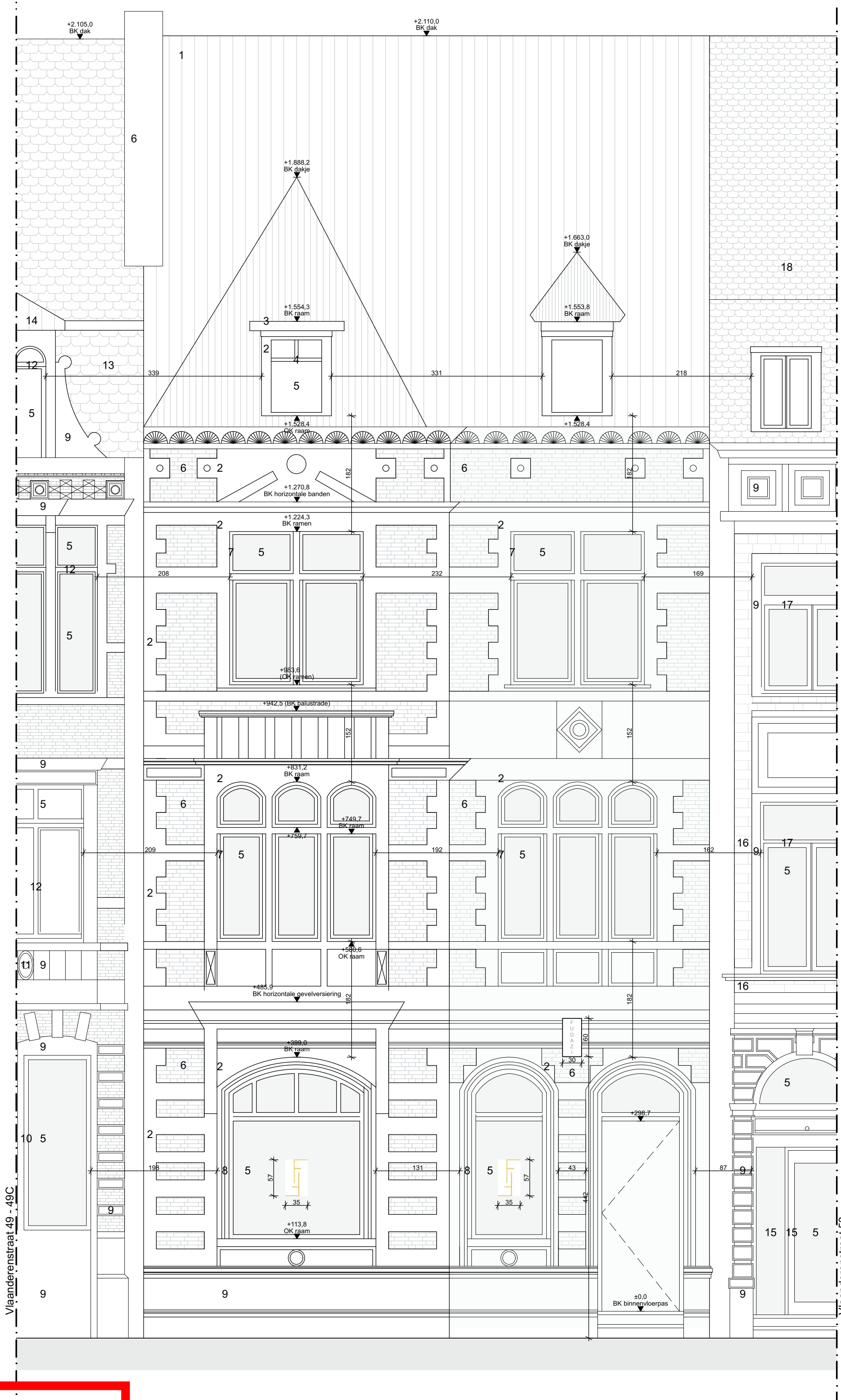
Voorgevel, nieuwe toestand Schaal 1/50
