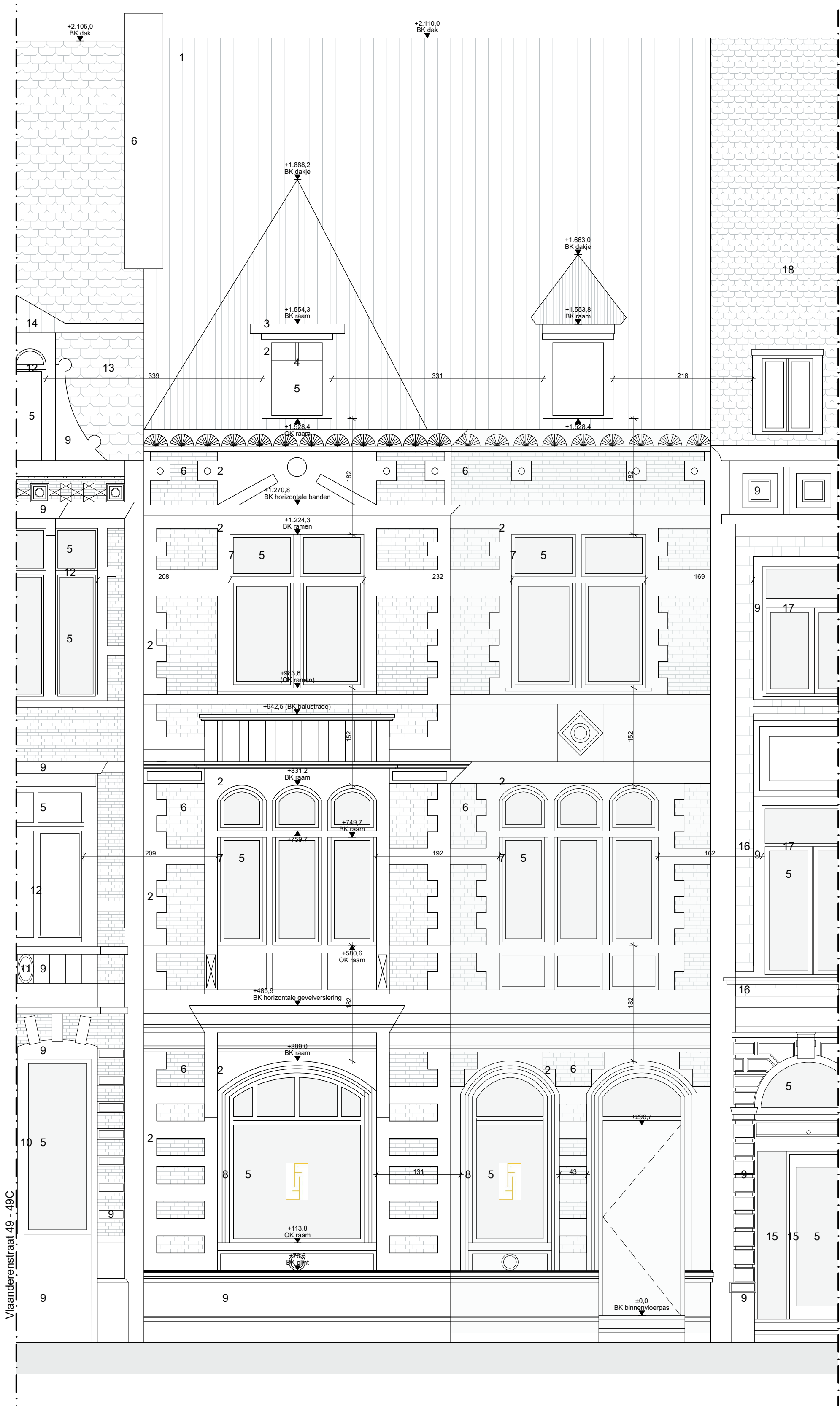
Voorgevel, bestaande toestand Schaal 1/50
