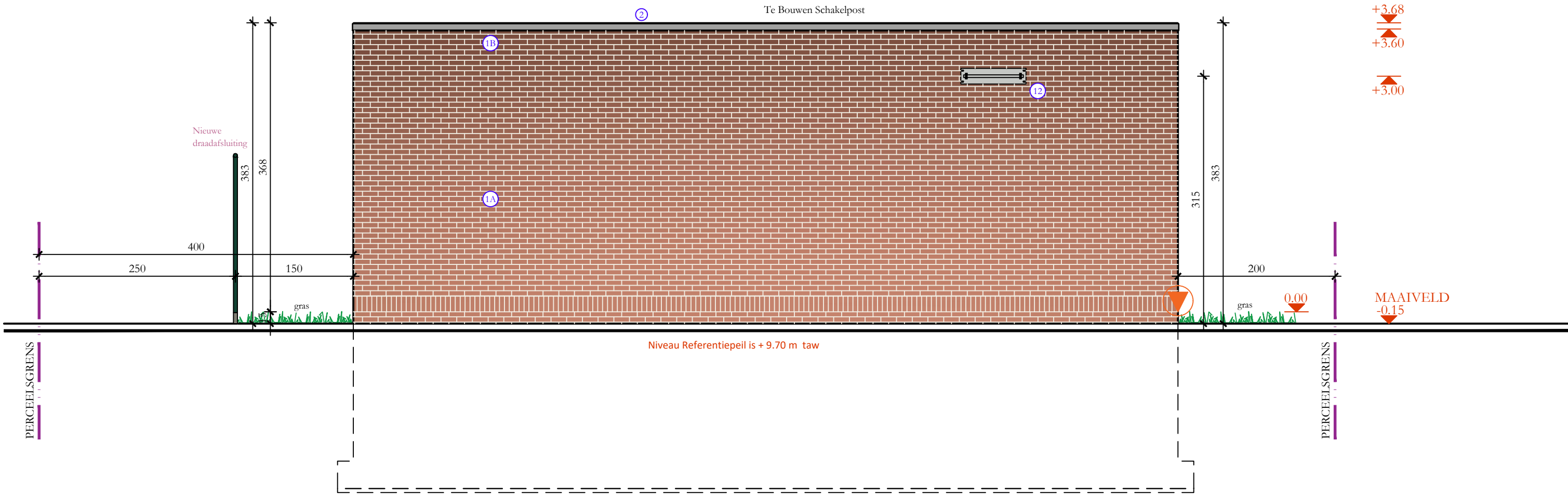
ZIJGEVEL LINKS OP SCHAAL 1 / 50 Meetlijn 0 1 2 3 4m
