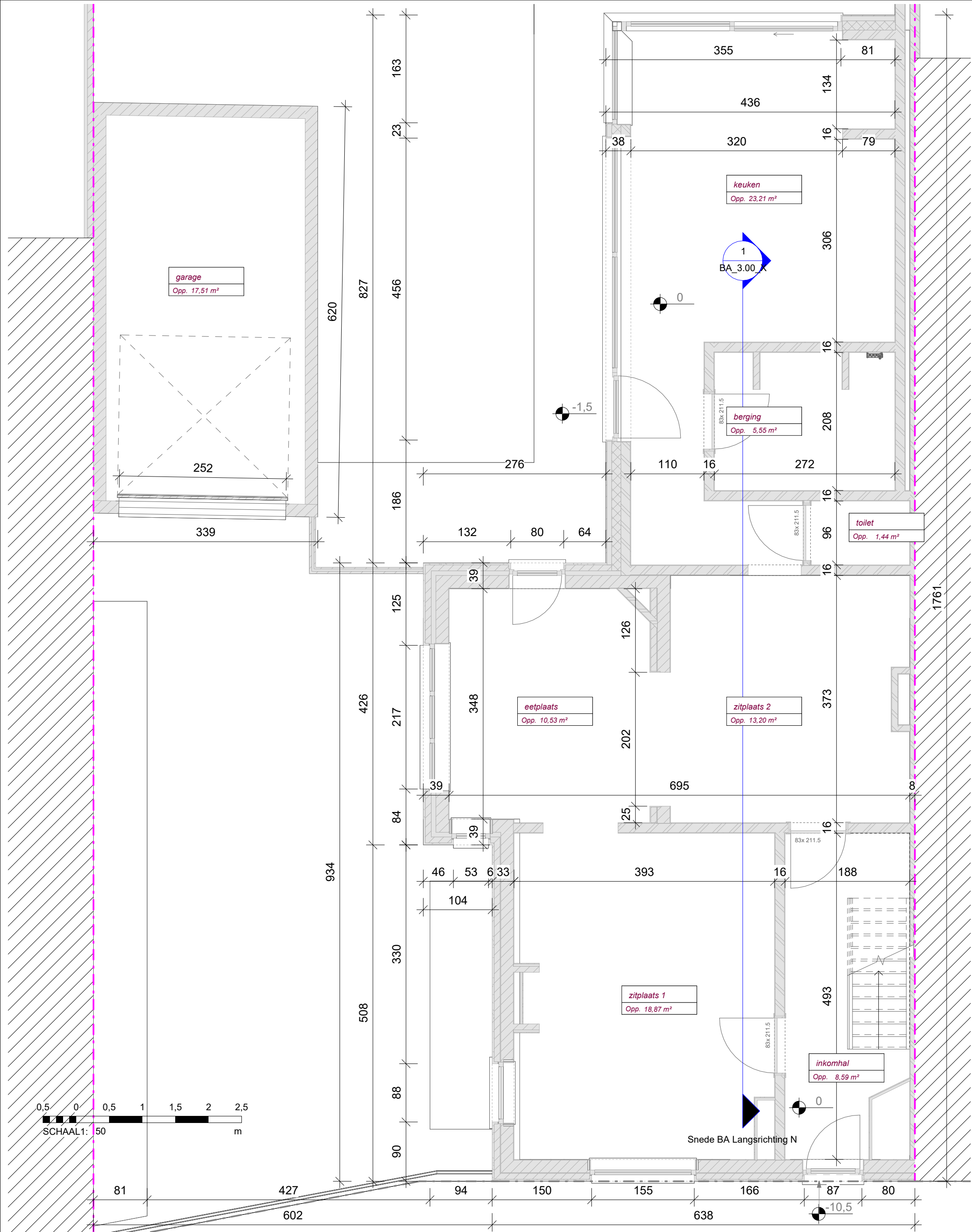
BA_1.00_X P_N_1.00_Grondplan Gelijkvloers
