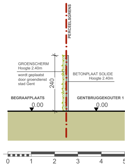
TERREINPROFIEL A - NIEUWE TOESTAND SCHAAL 1:100
