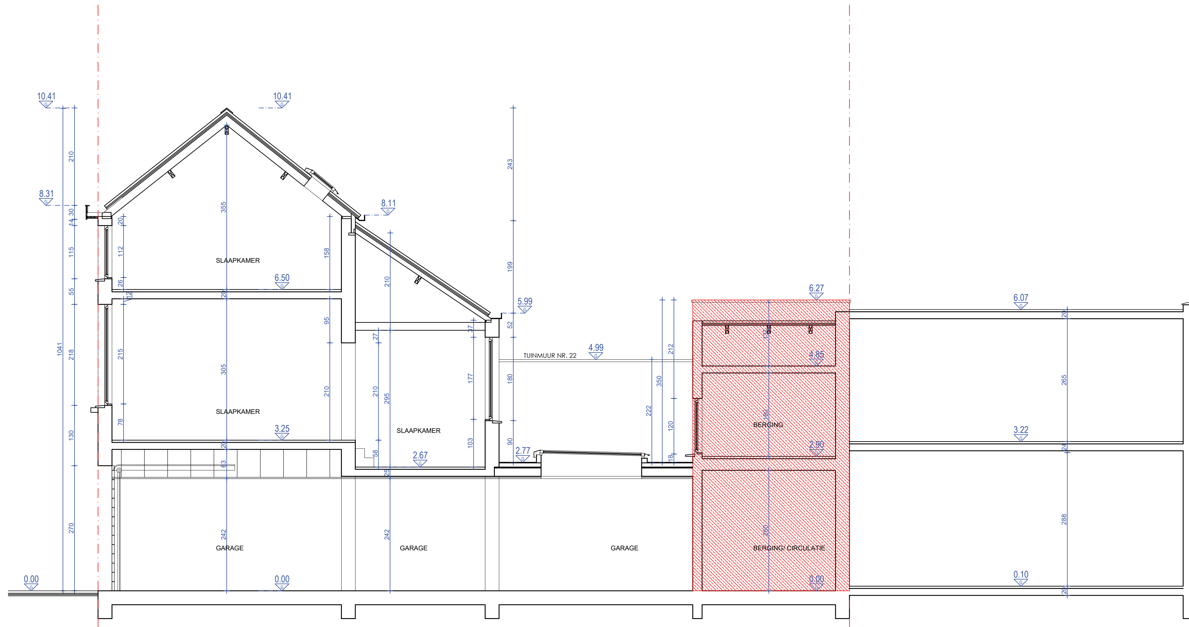
PRINCIPE DOORSNEDE bestaande toestand - schaal 1/50
