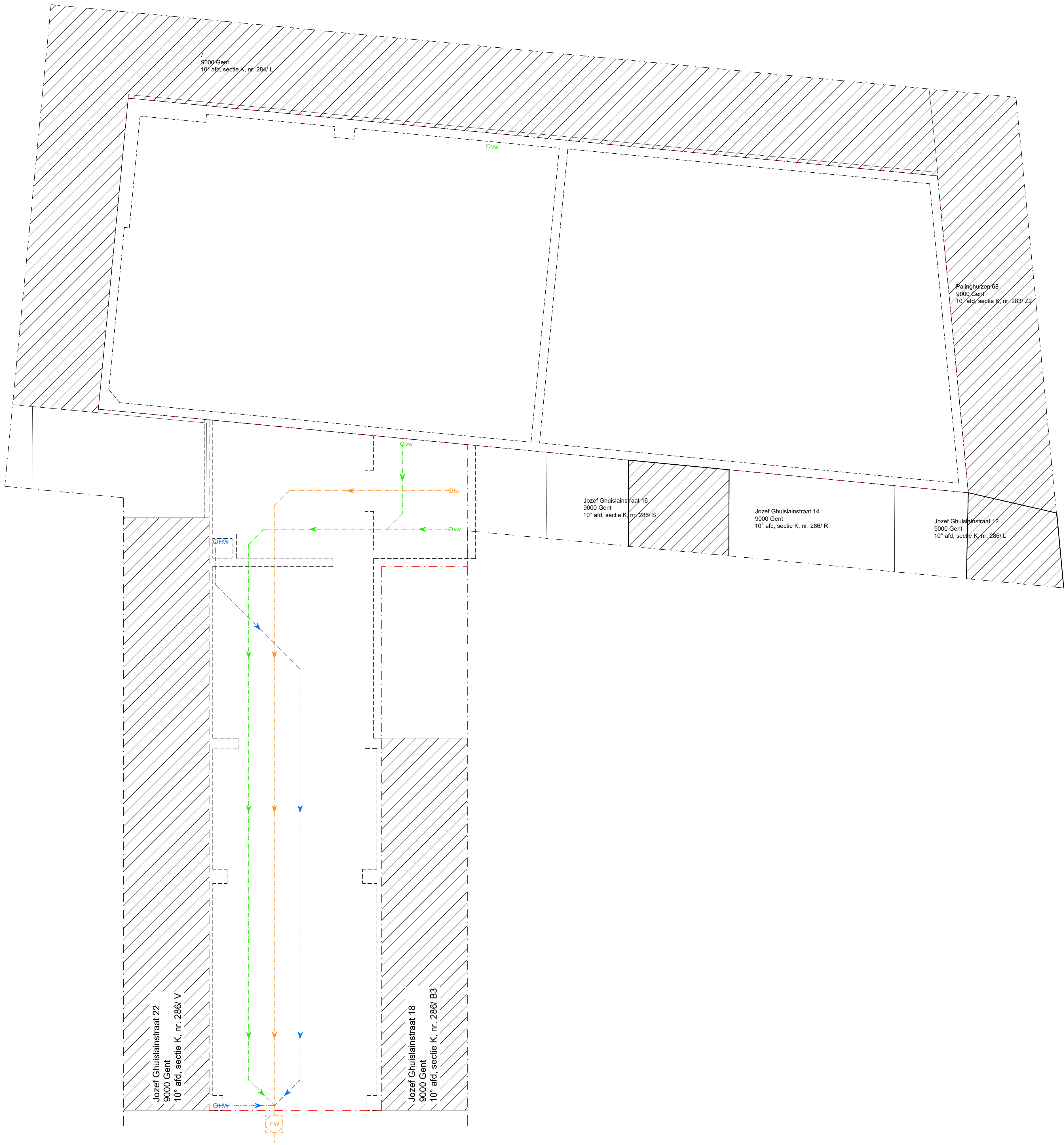
Gelijkvloers bestaande toestand - schaal 1/50
