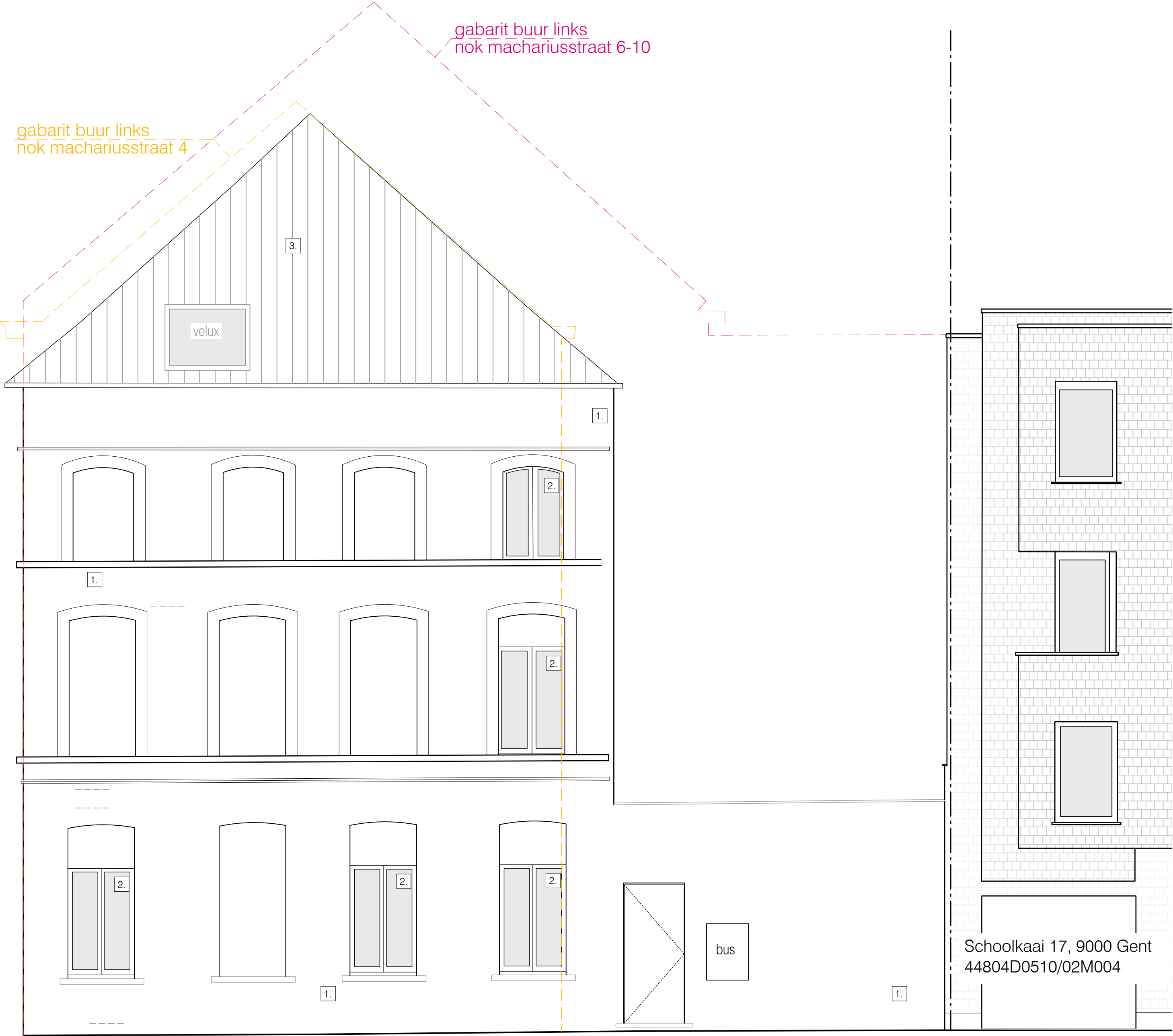
BESTAANDE TOESTAND VOORGEVEL (Schoolkaai) schaal: 1/50 - maatvoering in cm
