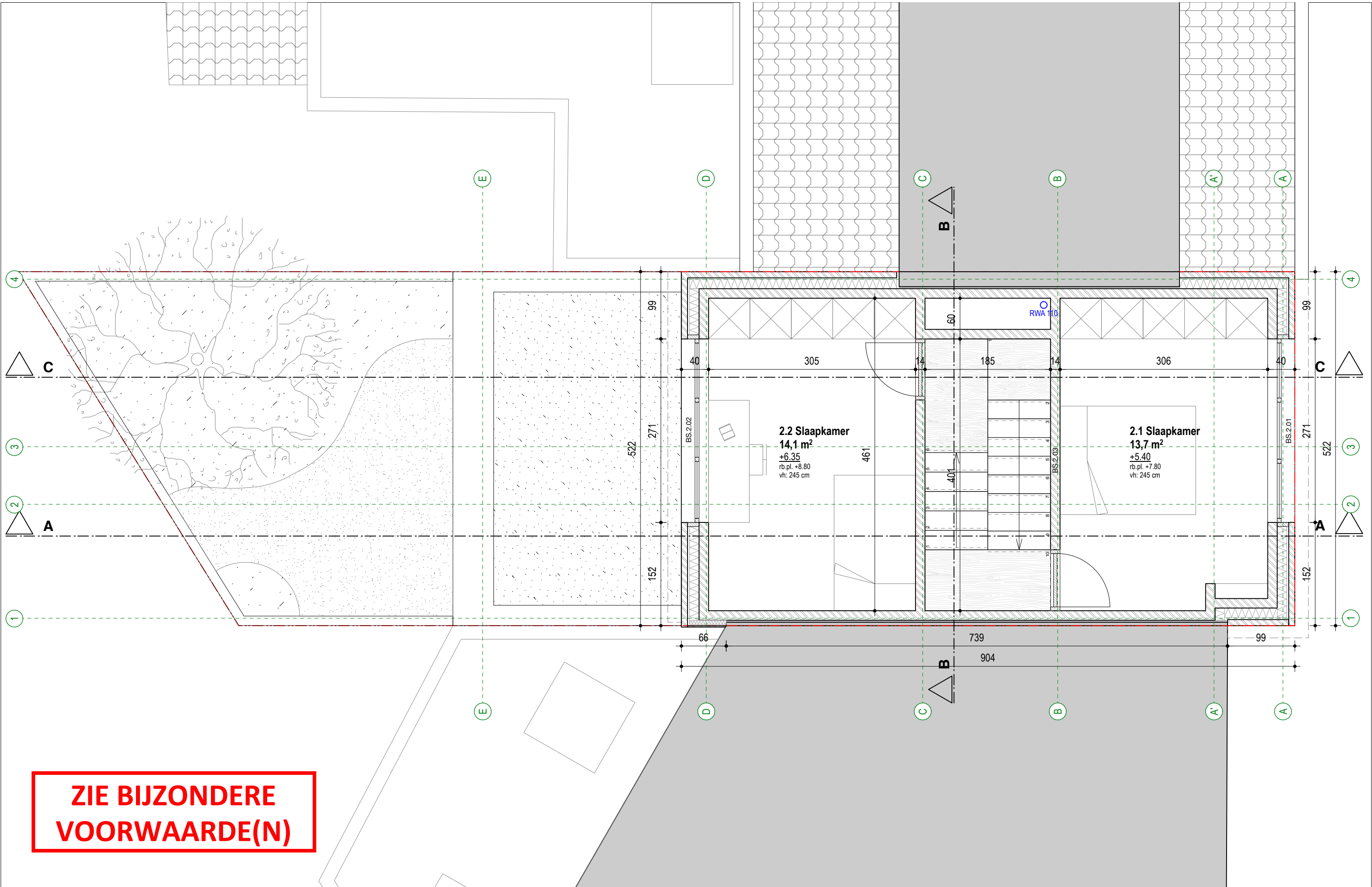
Grondplan +2 - nieuwe toestand
