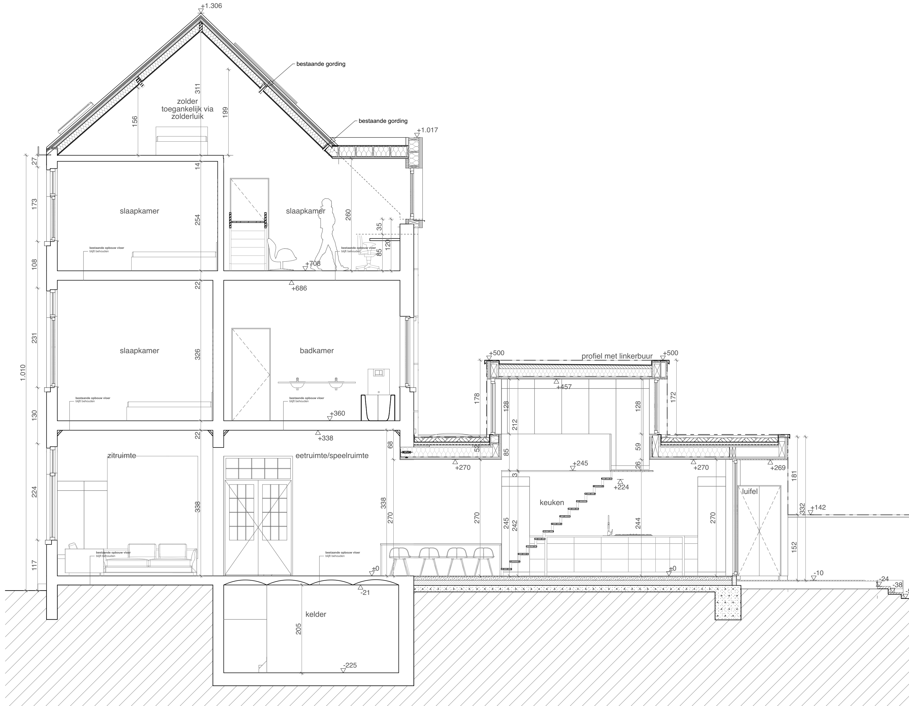
B Doorsnede B-B 1:50
