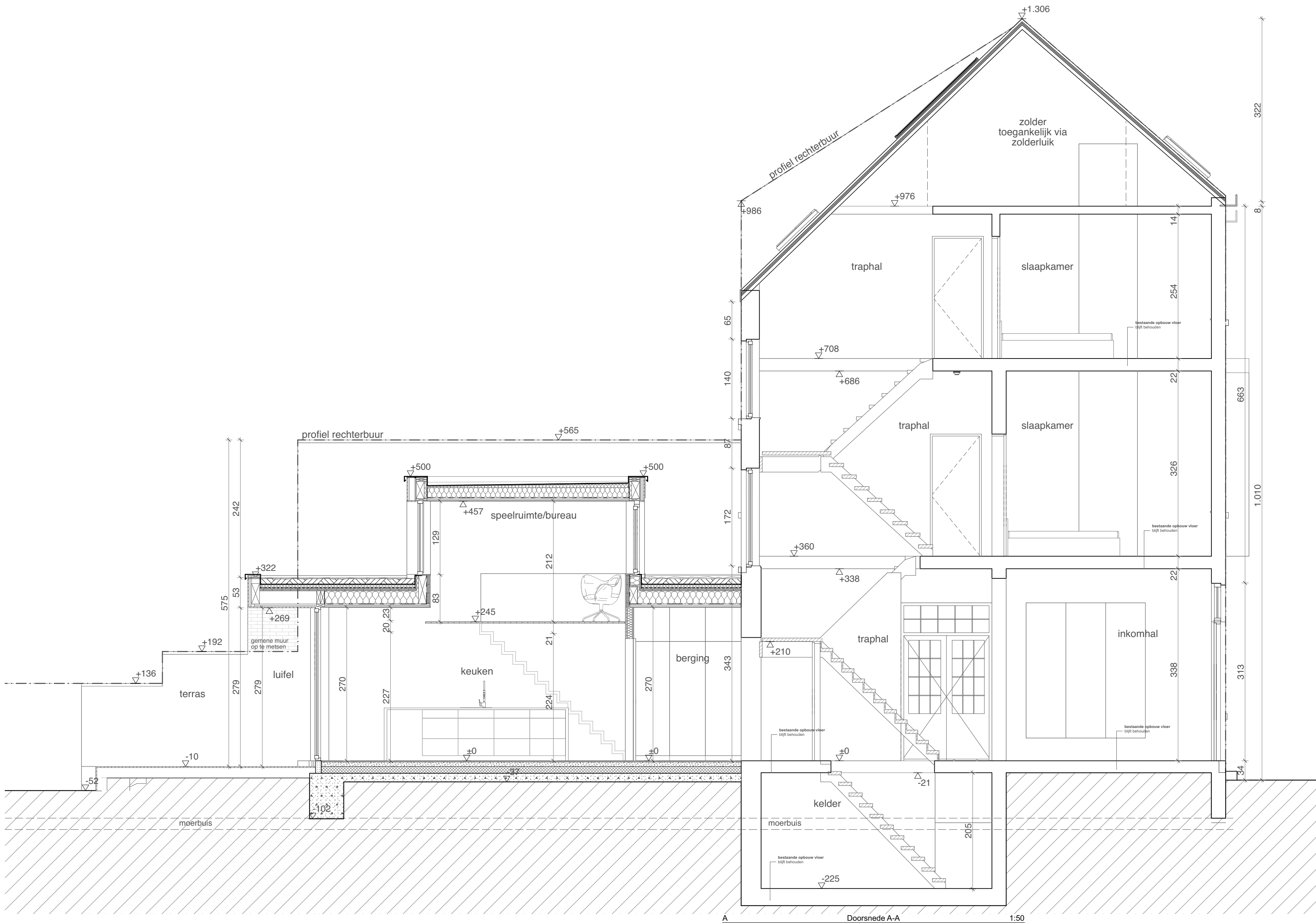
A Doorsnede A-A 1:50
