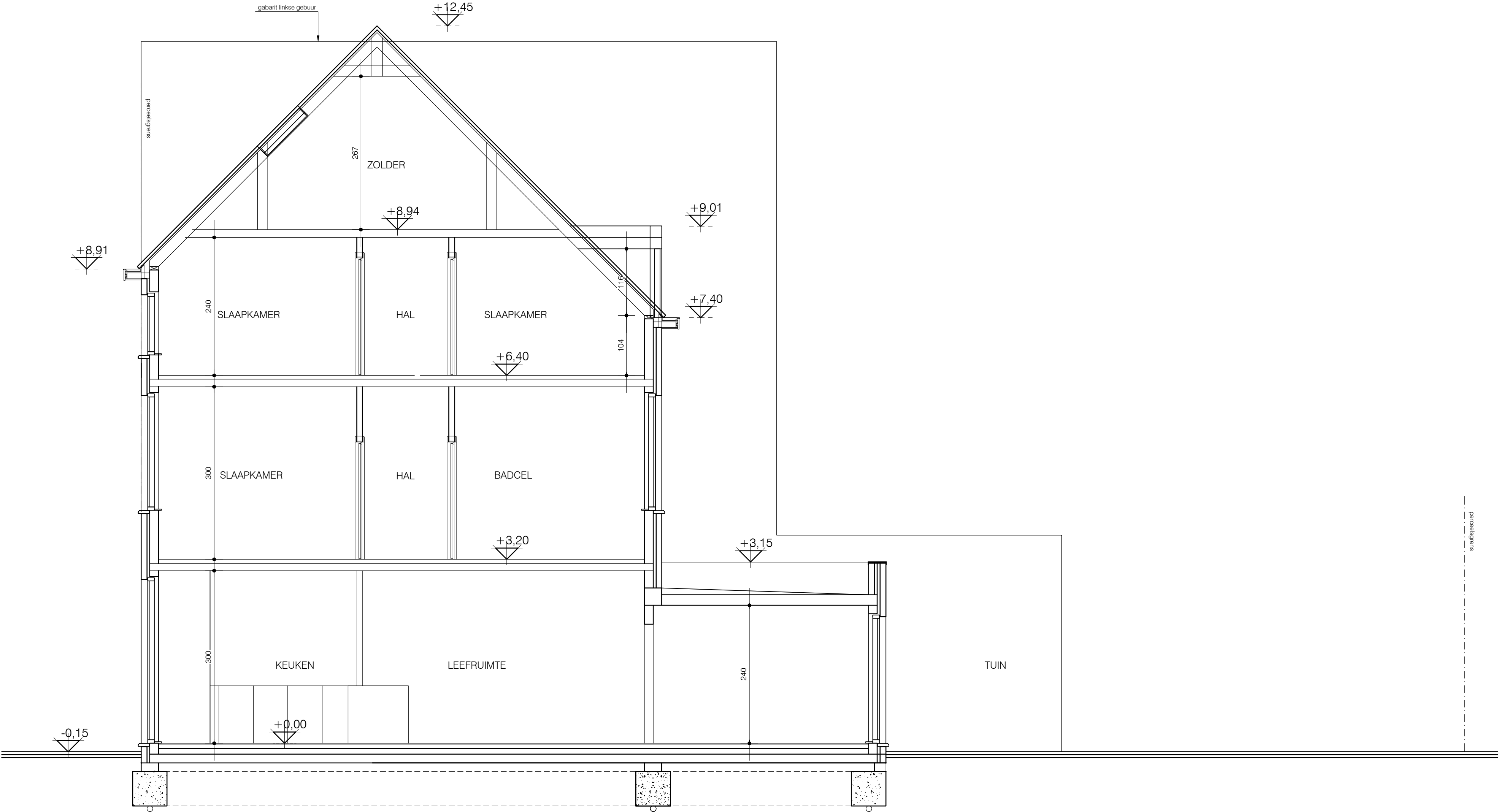
DOORSNEDE AA nieuwe (=bestaande) toestand alle afmetingen zijn in cm
