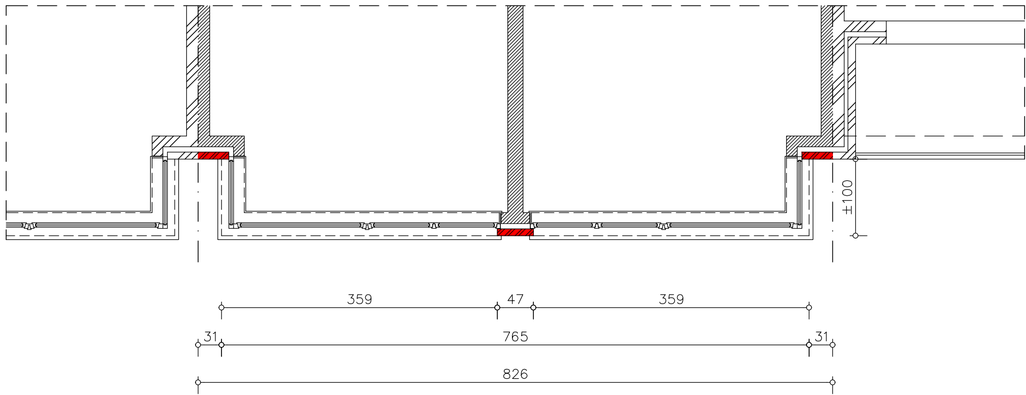
BESTAAND PLAN 5de VERDIEPING Niv +14.00
