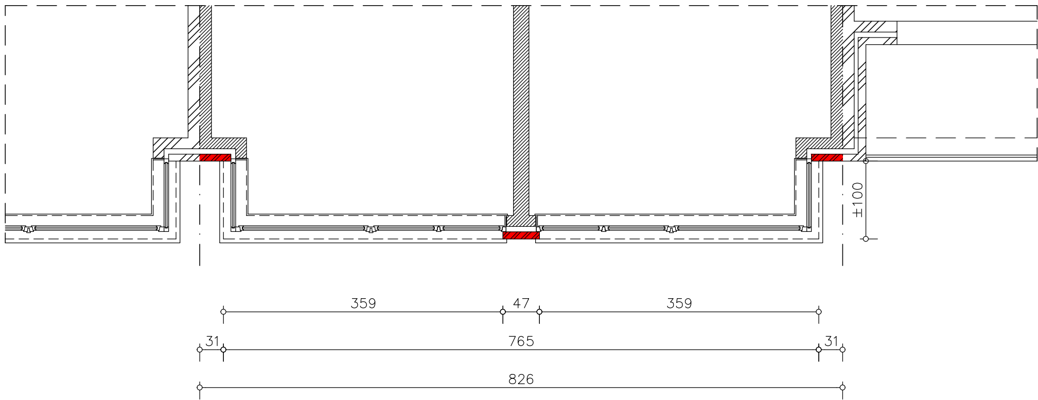
BESTAAND PLAN 4de VERDIEPING Niv +11.20
