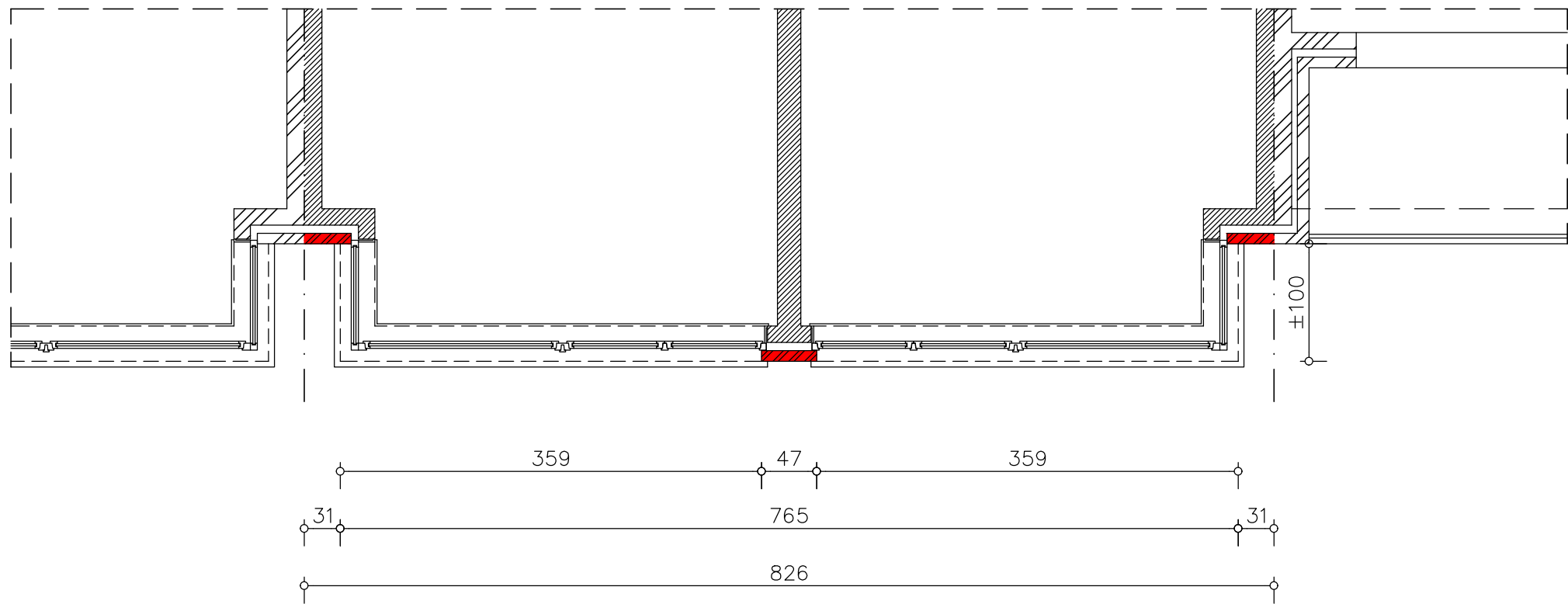
BESTAAND PLAN 2de VERDIEPING Niv +5.60 .
