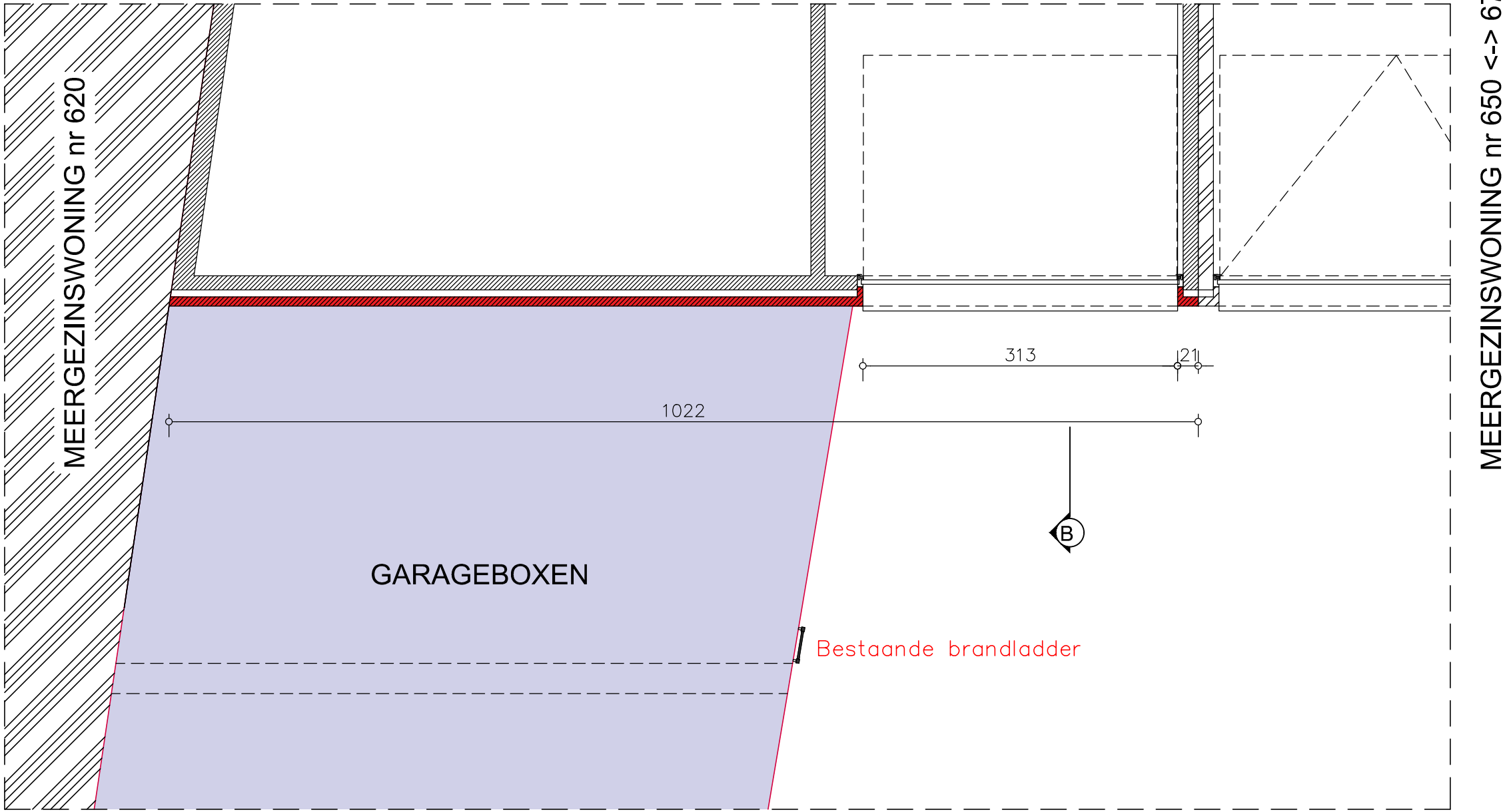
BESTAAND GRONDPLAN Niv 0.00 .
