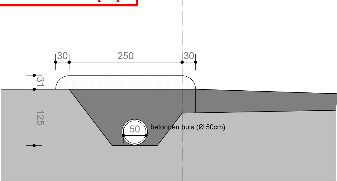
Dwarse snede
