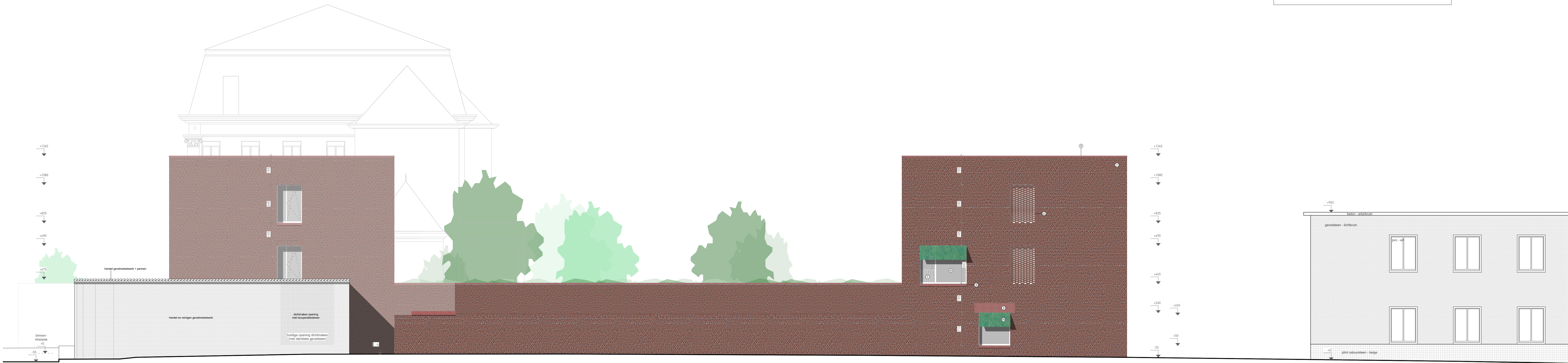
GEVEL 1 - VOORGEVEL
