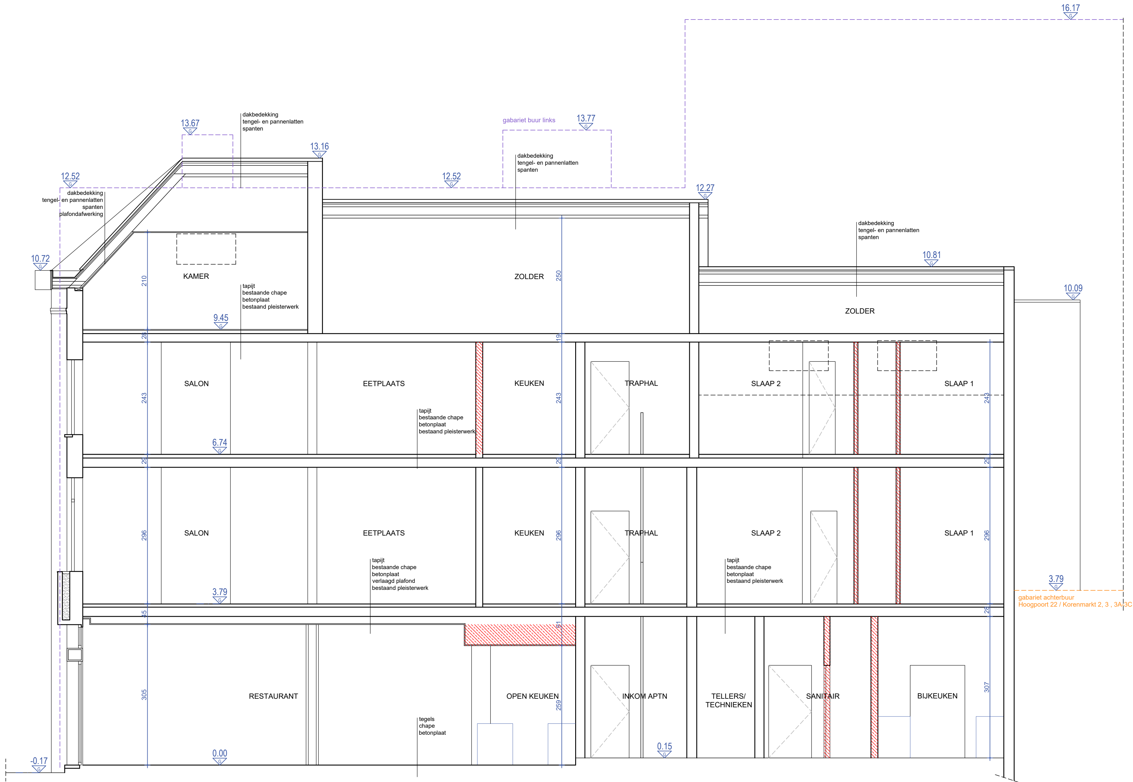
SNEDE B bestaande toestand schaal 1:50
