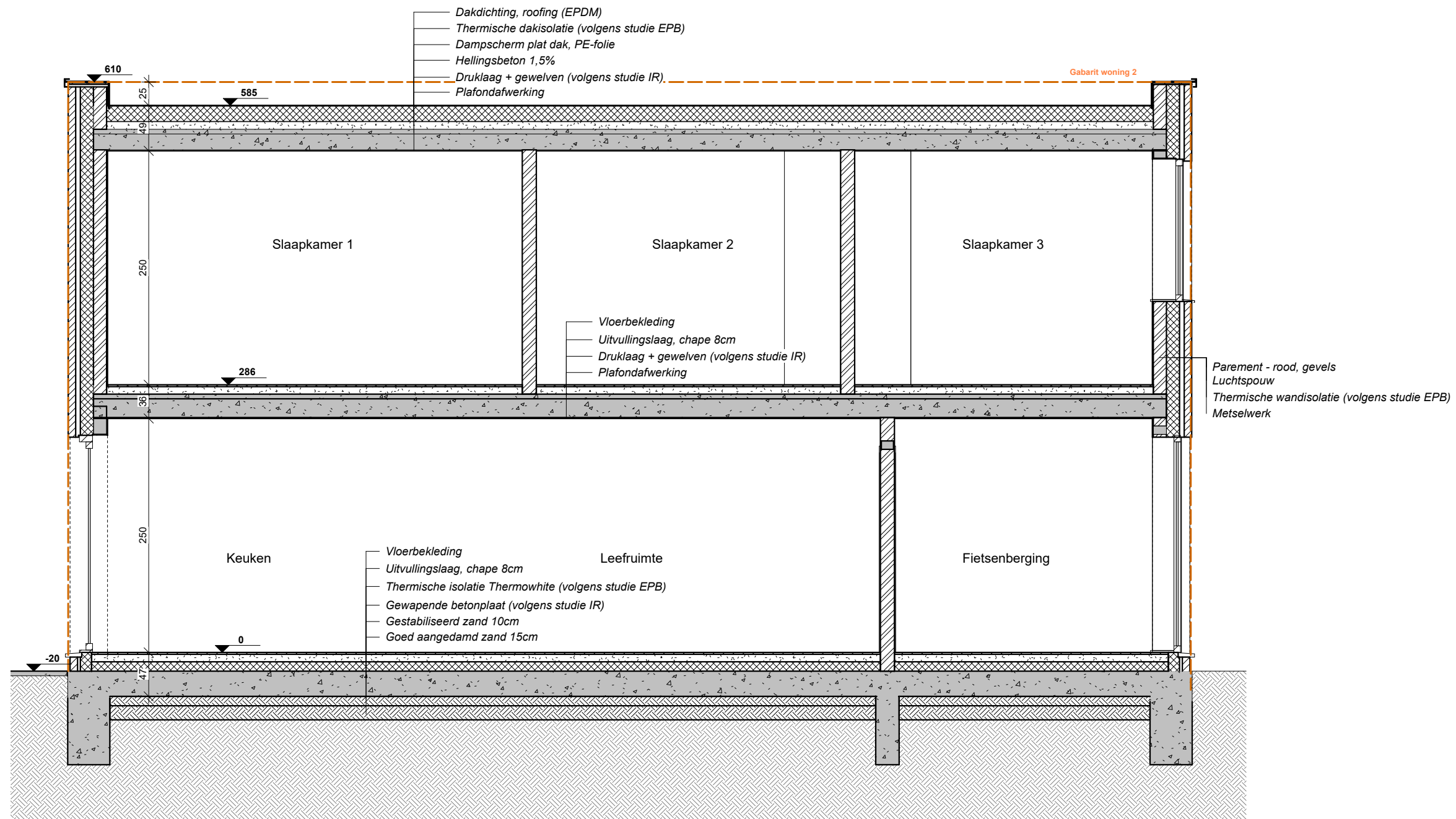
WONING 1
