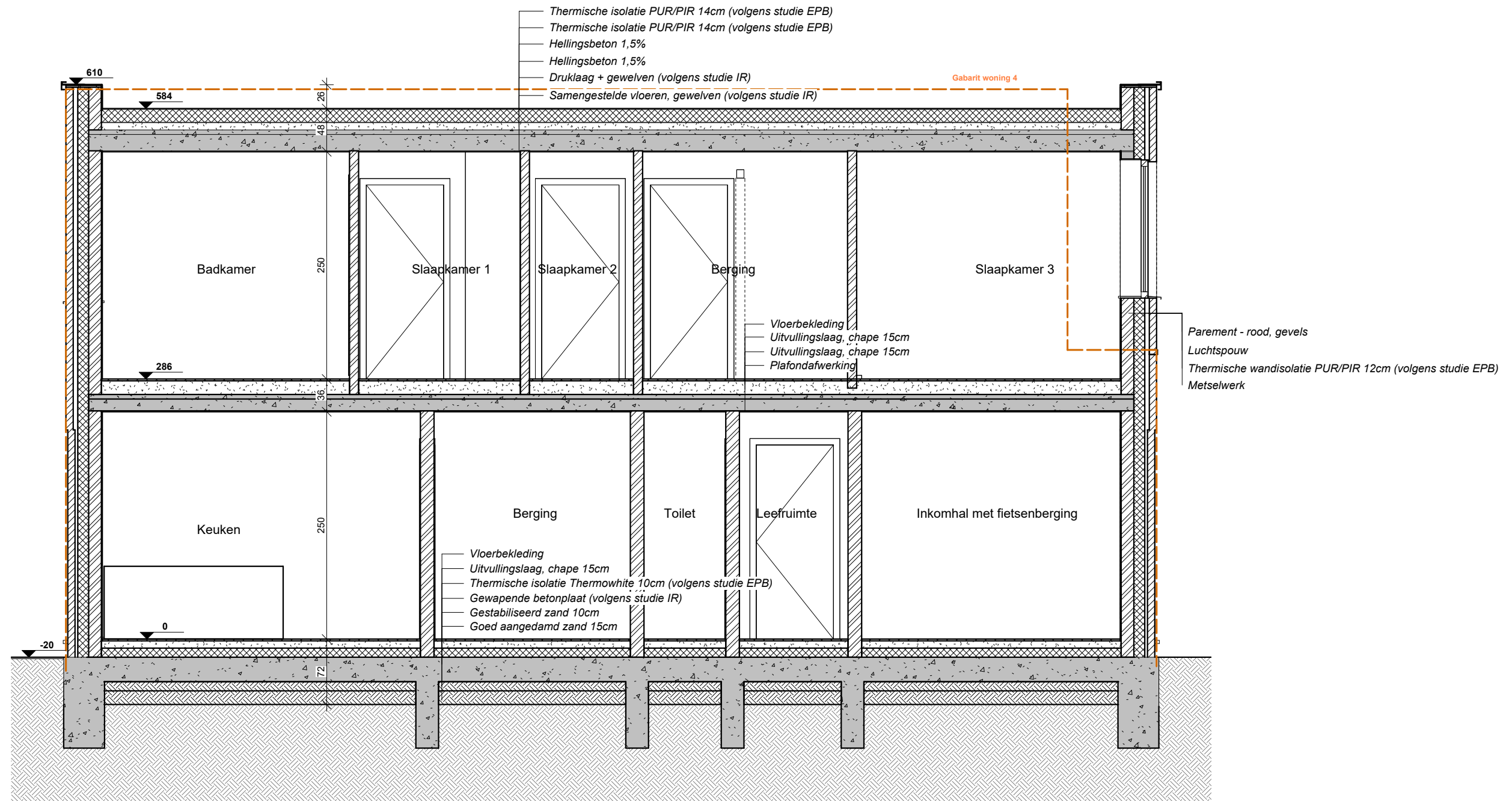
WONING 3
