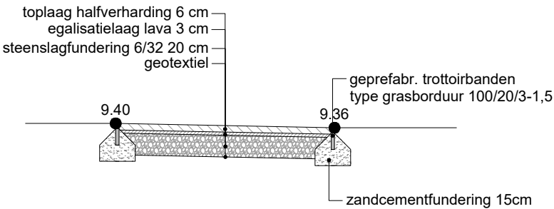
type dwarsprofiel 07 dwarsprofiel parkpad binnentuin schaal 1:50
