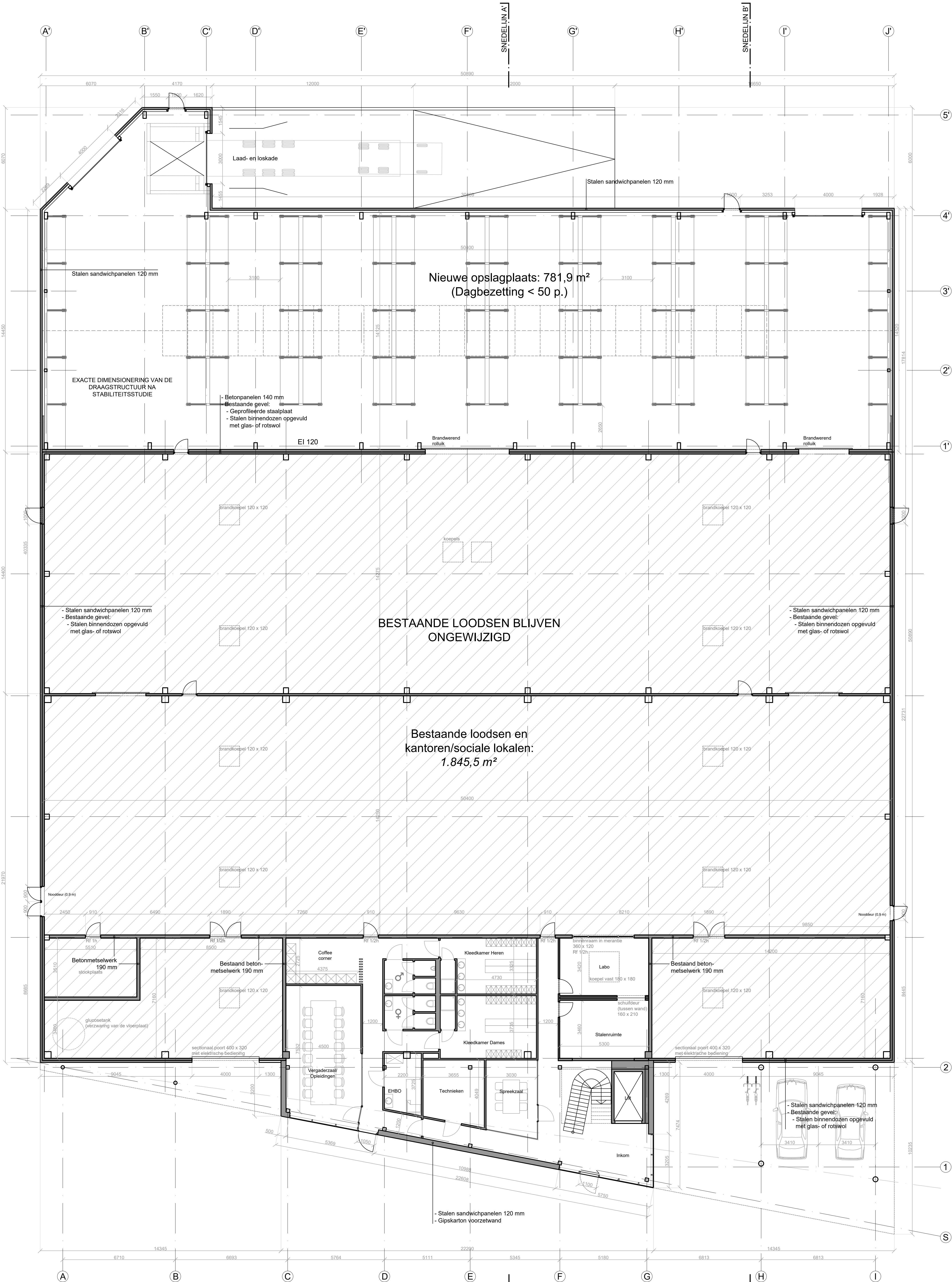
PLAN GELIJKVLOERS Nieuwe situatie
