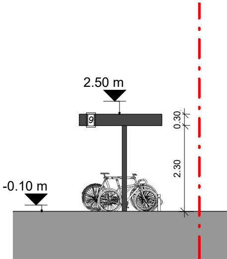
Rechterzijgevel fietsenstalling 1 : 100
