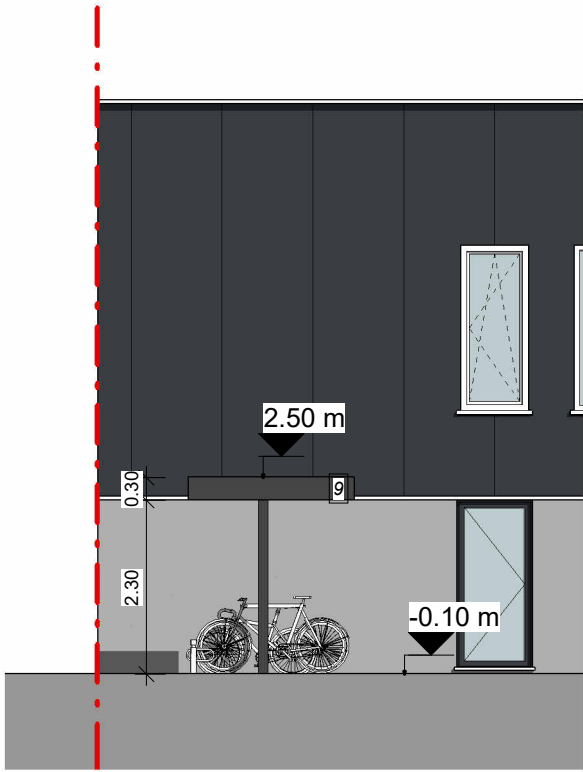
Linkerzijgevel fietsenstalling 1 : 100 0 1 2 3 4 5
