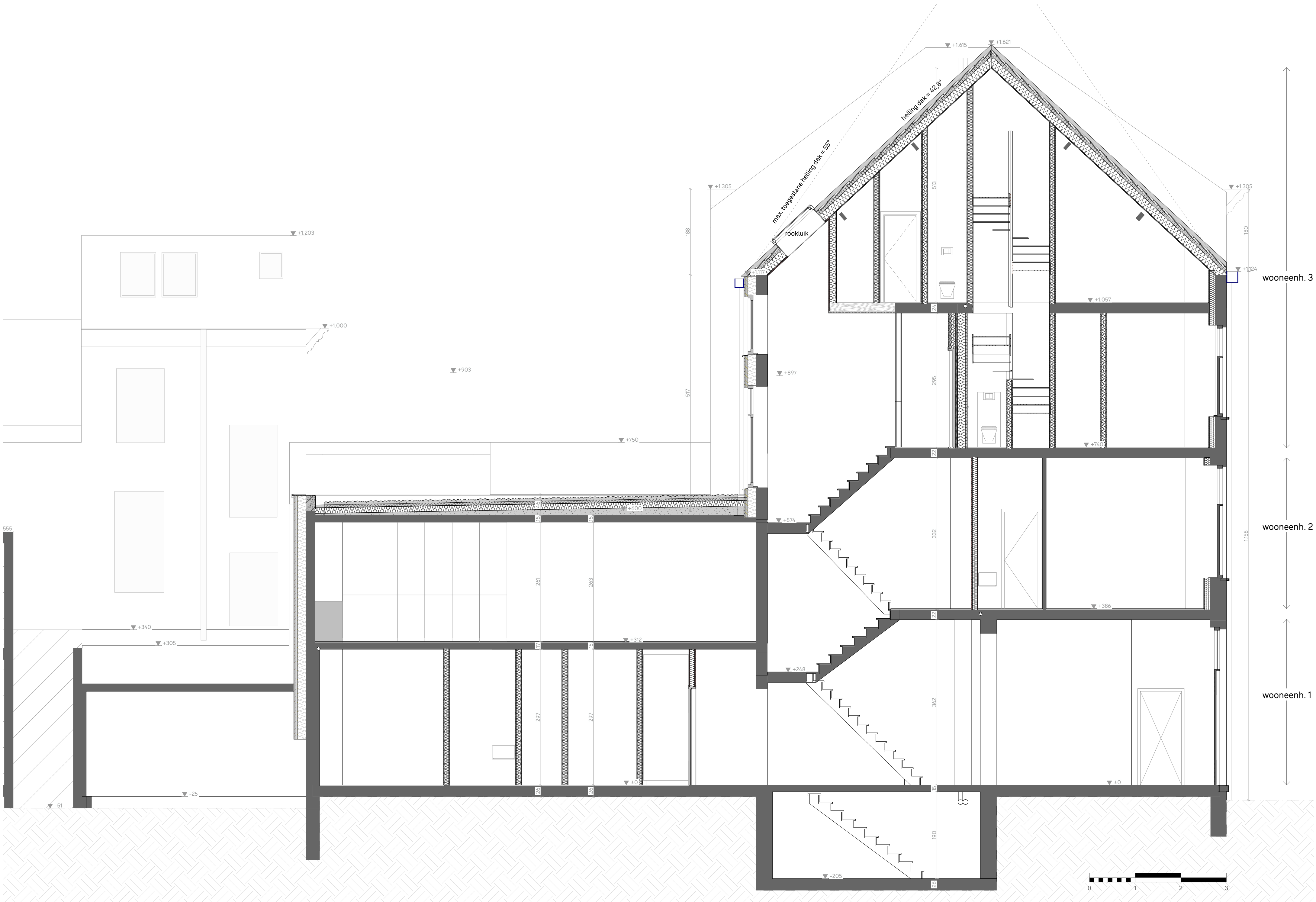
Doorsnede C-C
