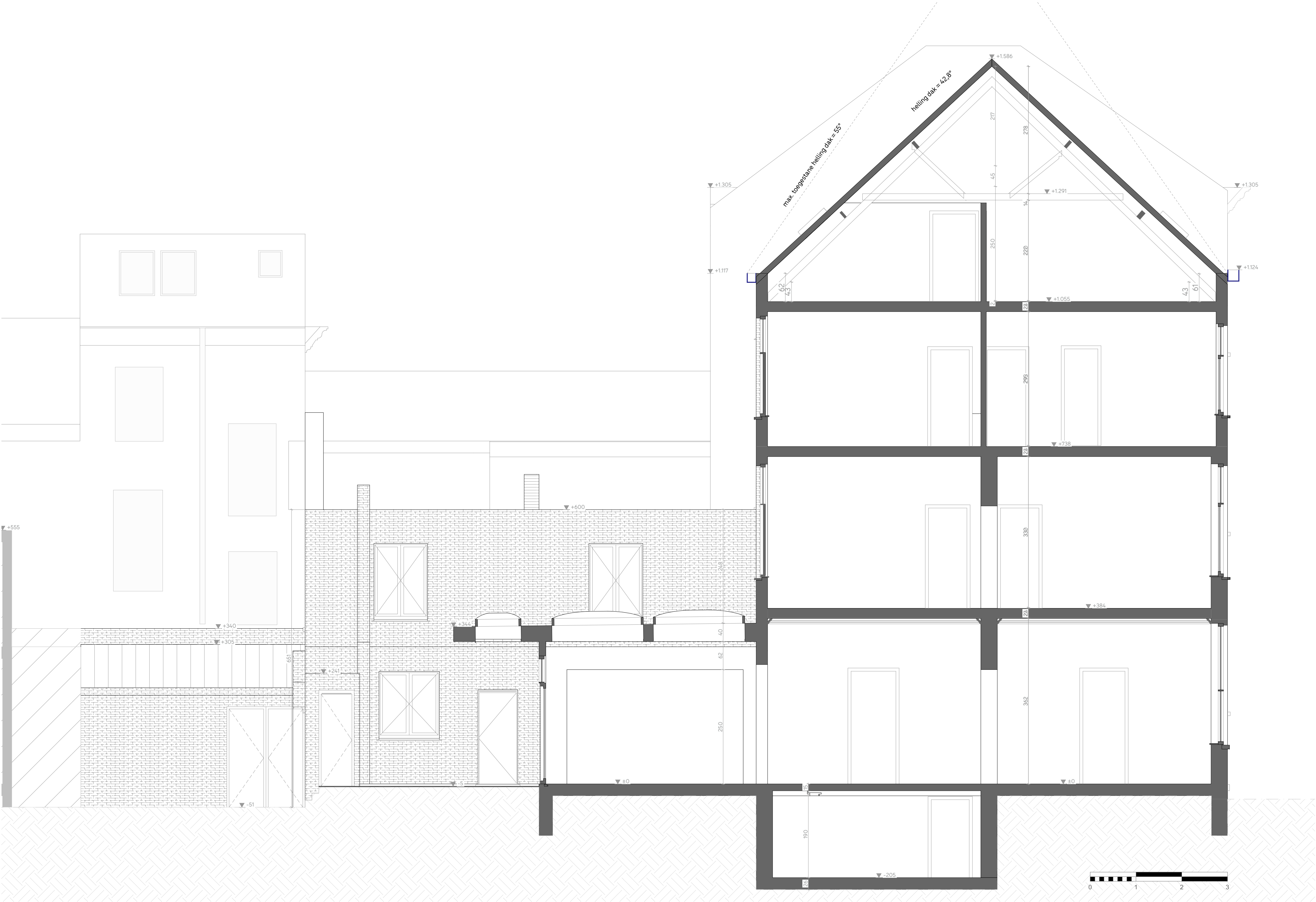
Doorsnede B-B
