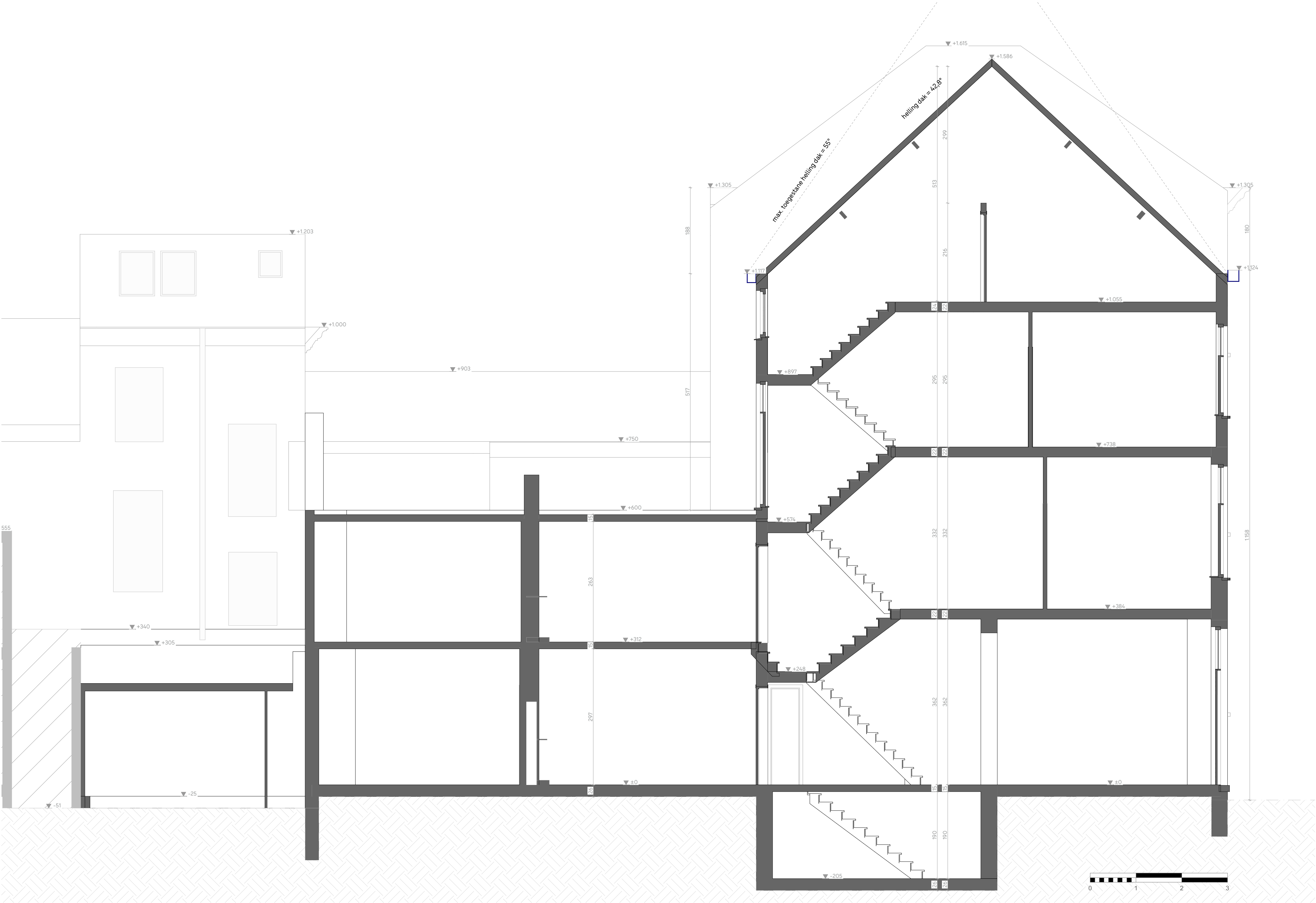
Doorsnede C-C
