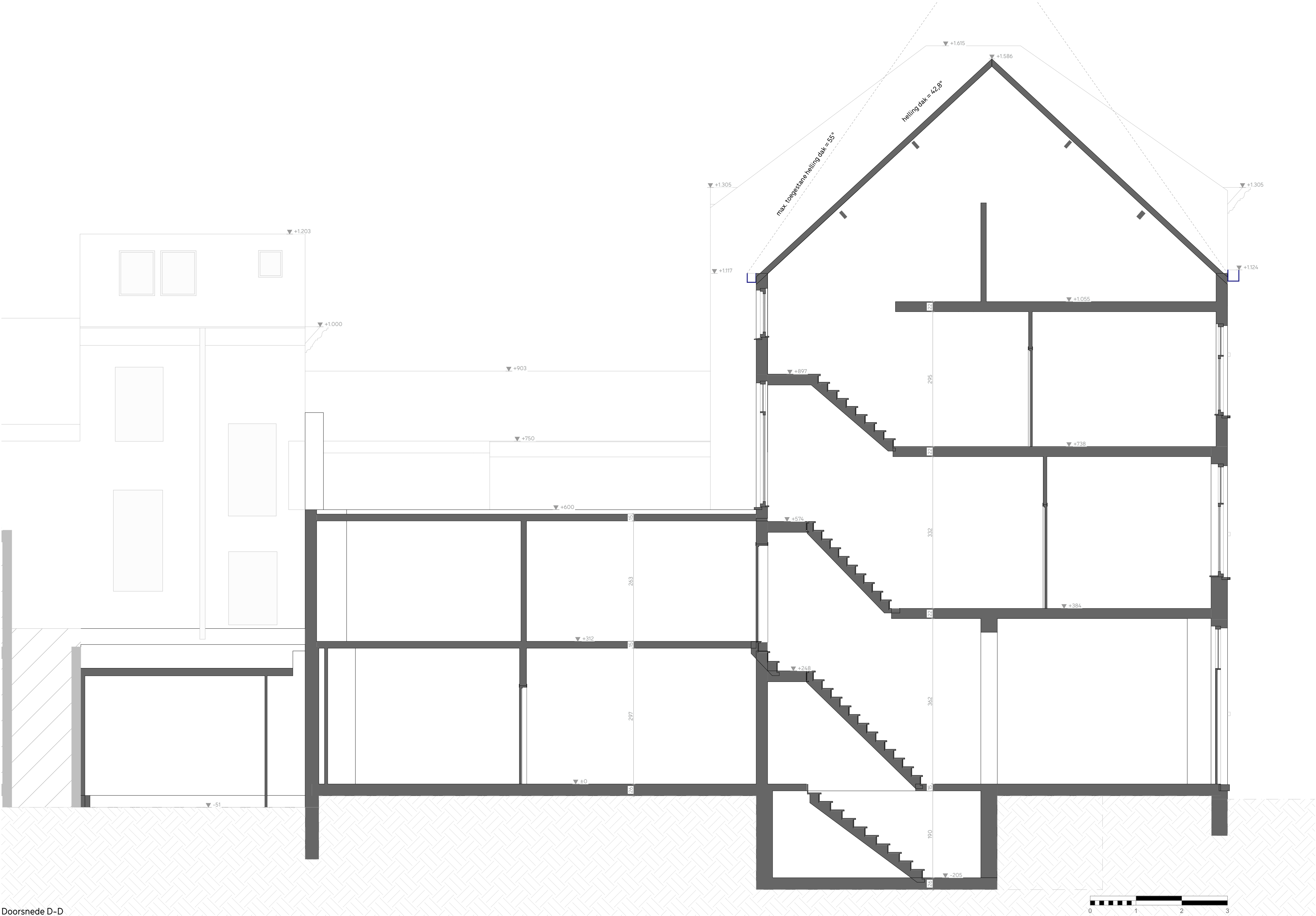
Doorsnede D-D
