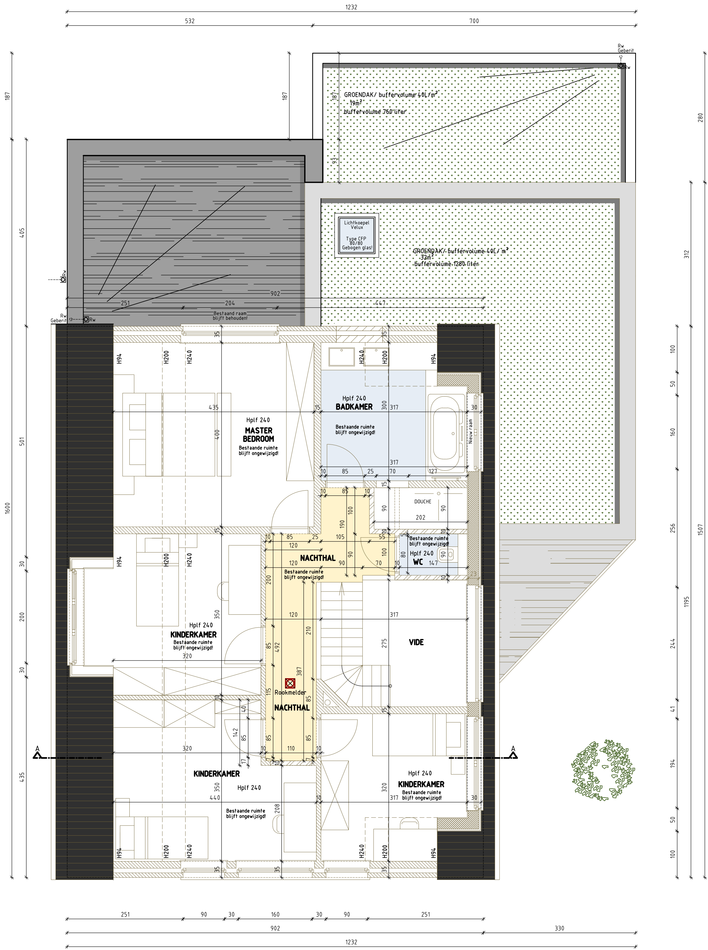
PLAN VERDIEPING 01 1/50 NIEUWE TOESTAND
