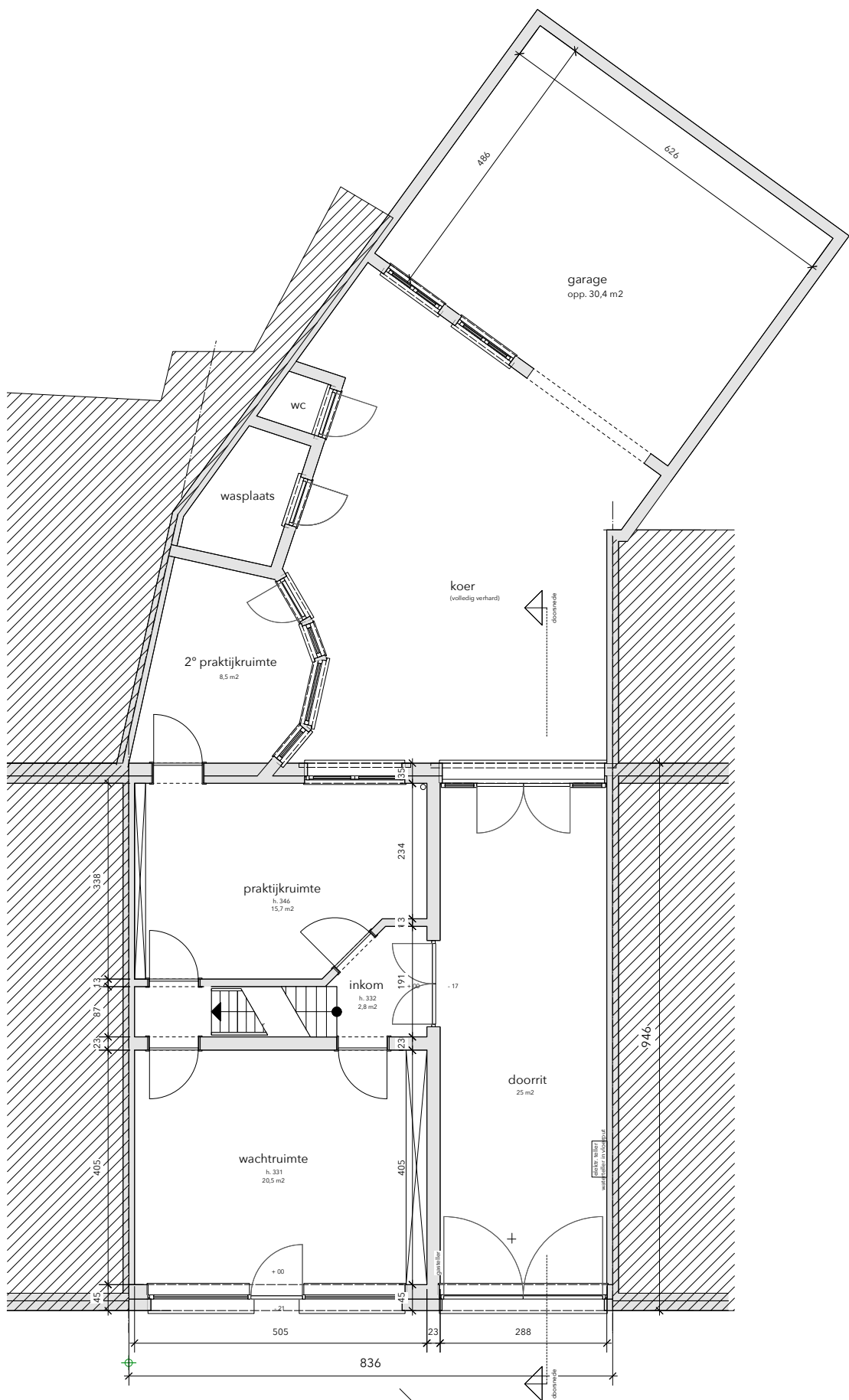
plan gelijkvloers
