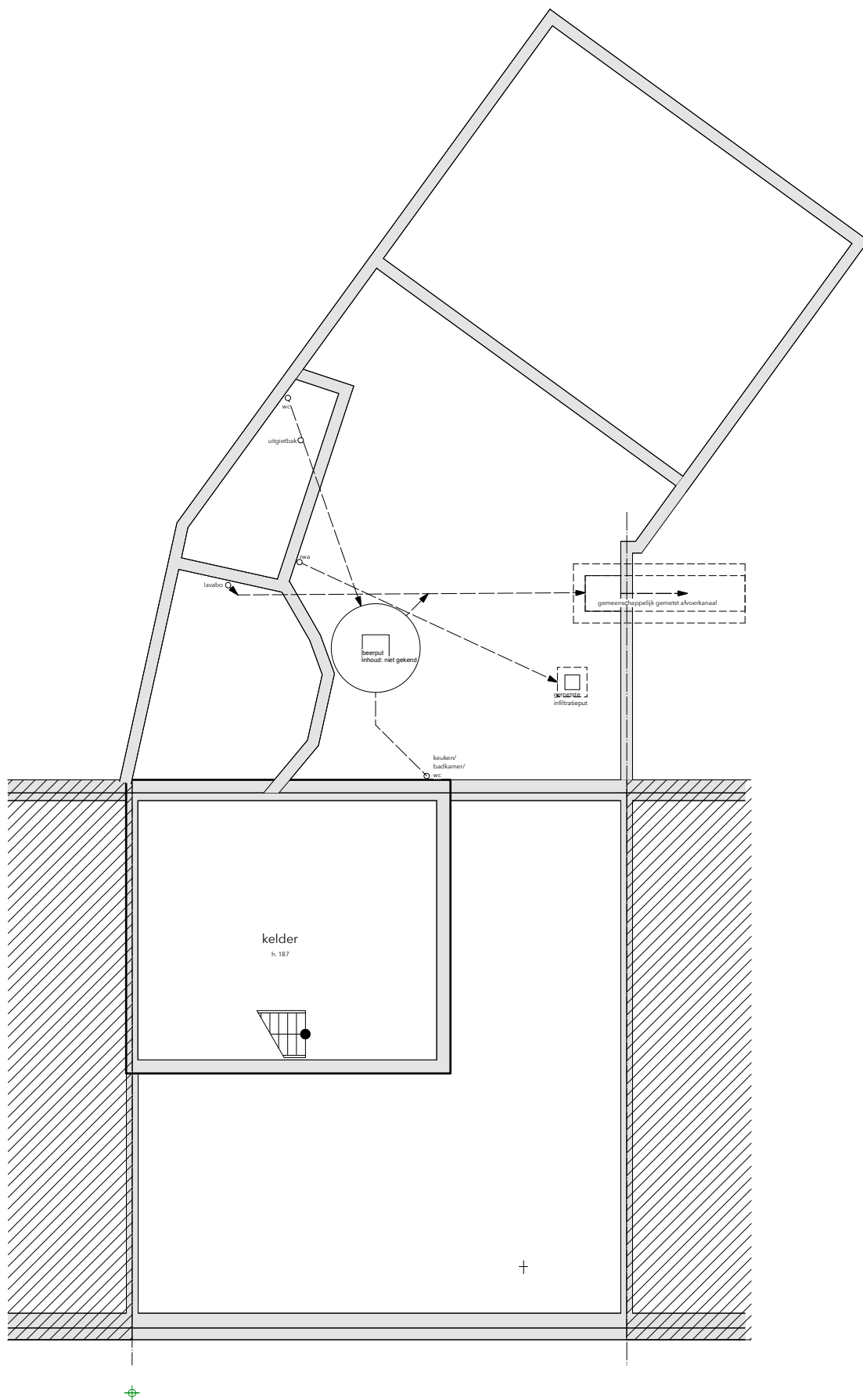
plan kelder, fundering en riolering
