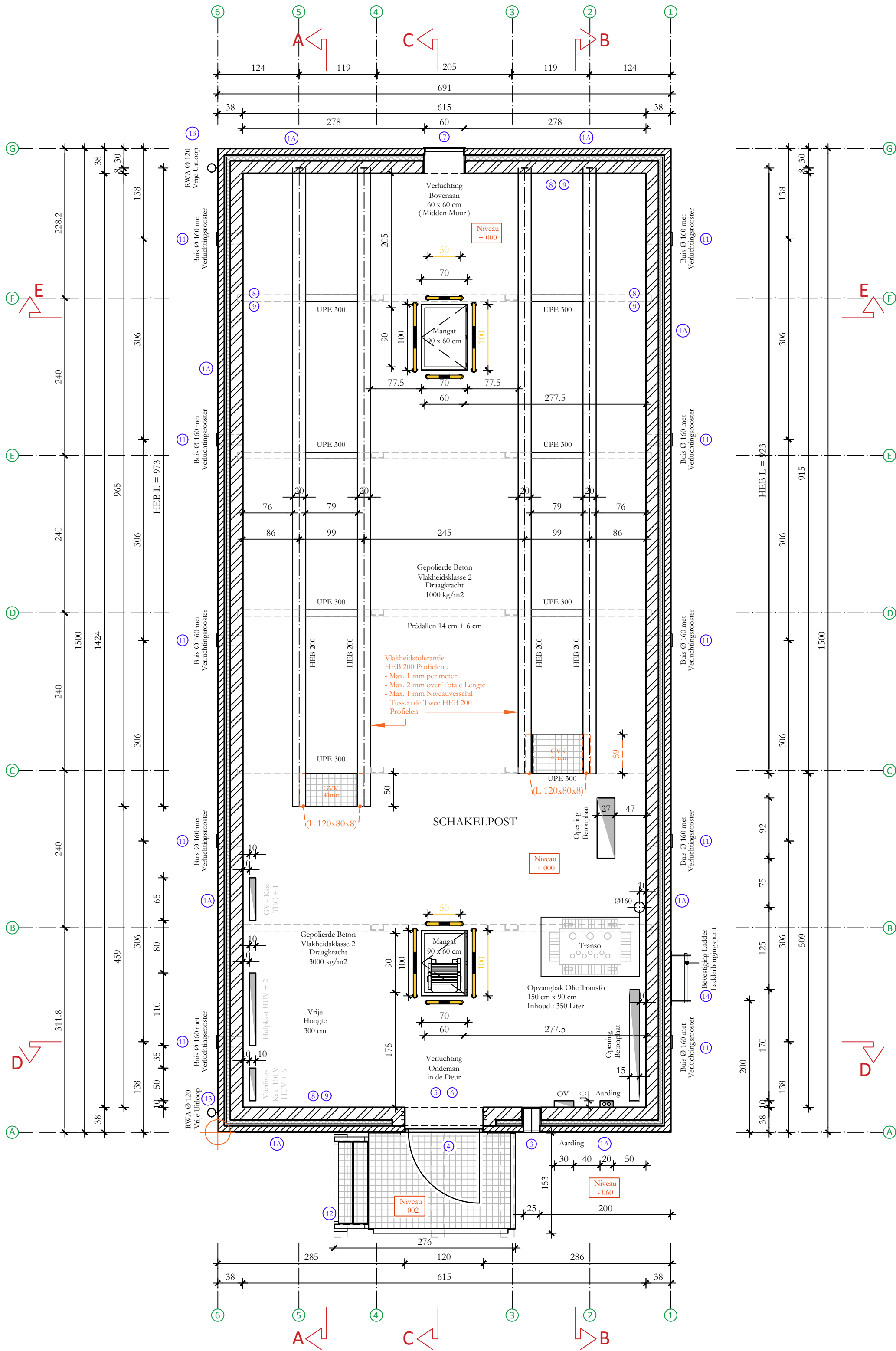
GRONDPLAN OP SCHAAL 1 / 50
