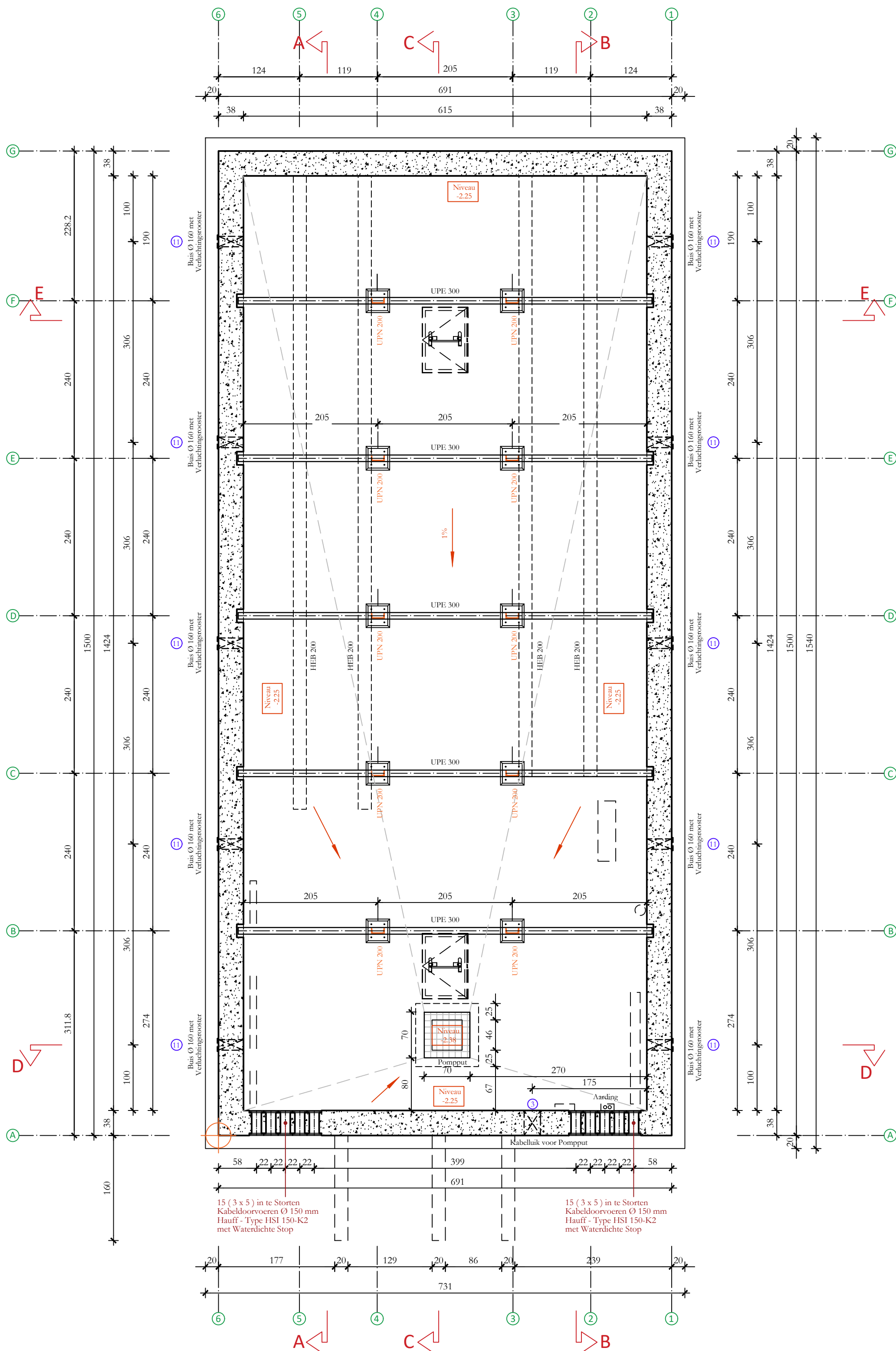
FUNDERINGSPLAN OP SCHAAL 1/ 50
