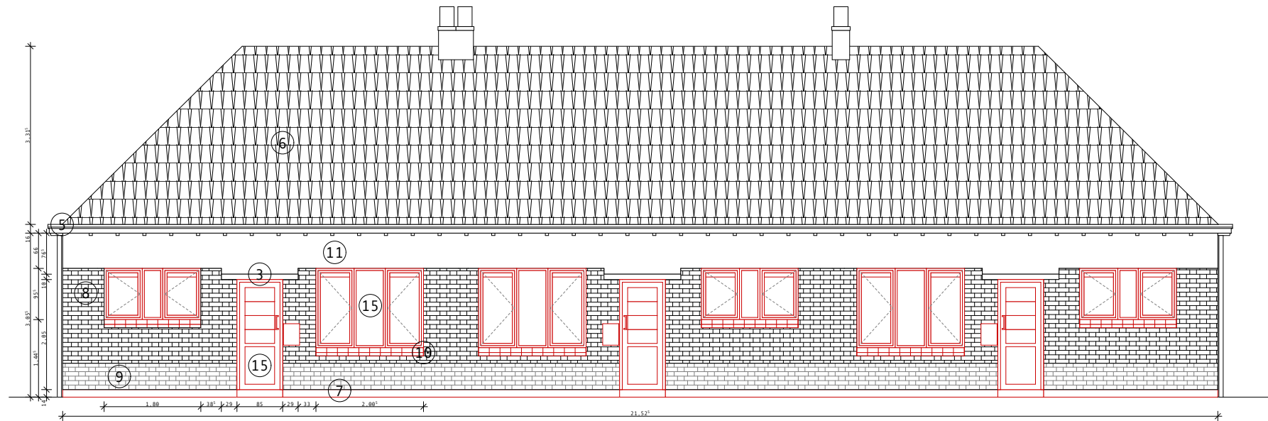
TYPE met 3 units, ramen hoog blok 1 + blok 5
