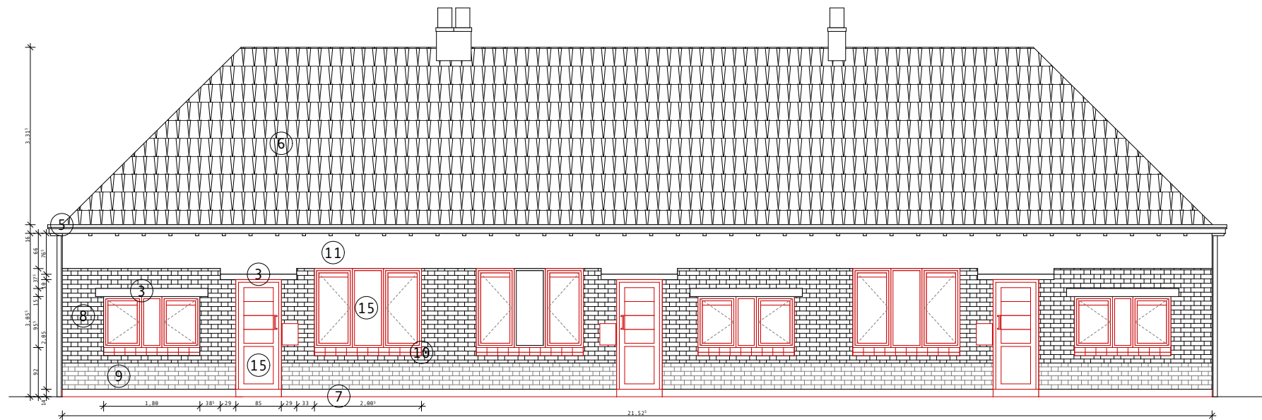
TYPE met 3 units, ramen laag blok 2 + blok 3
