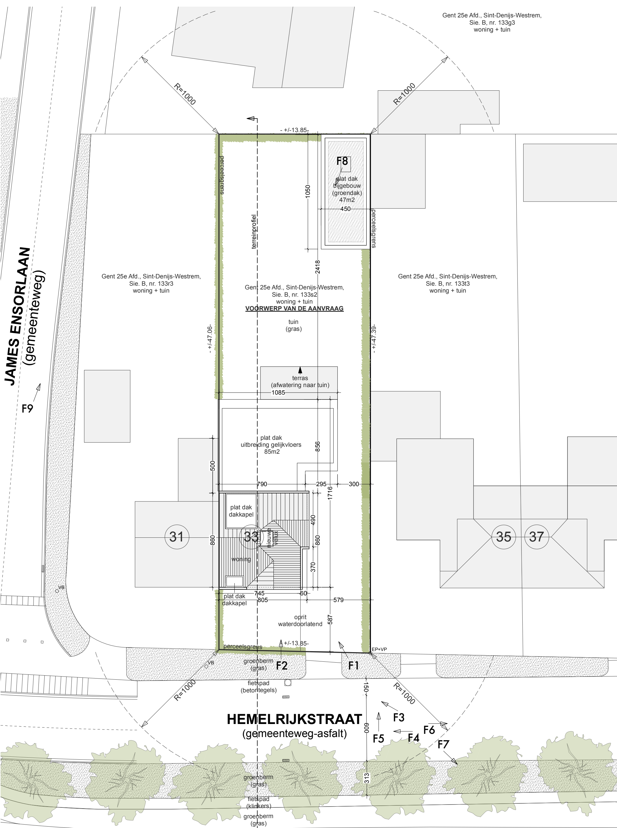
INPLANTINGSPLAN - VERGUNDE TOESTAND - SCHAAAL 1/200
