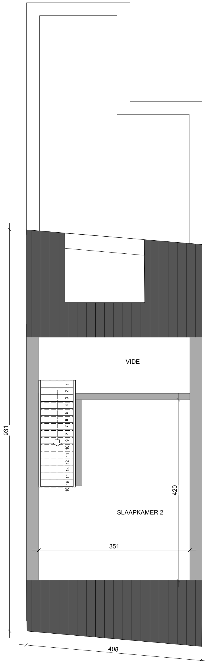
ZOLDER schaal 1/50
