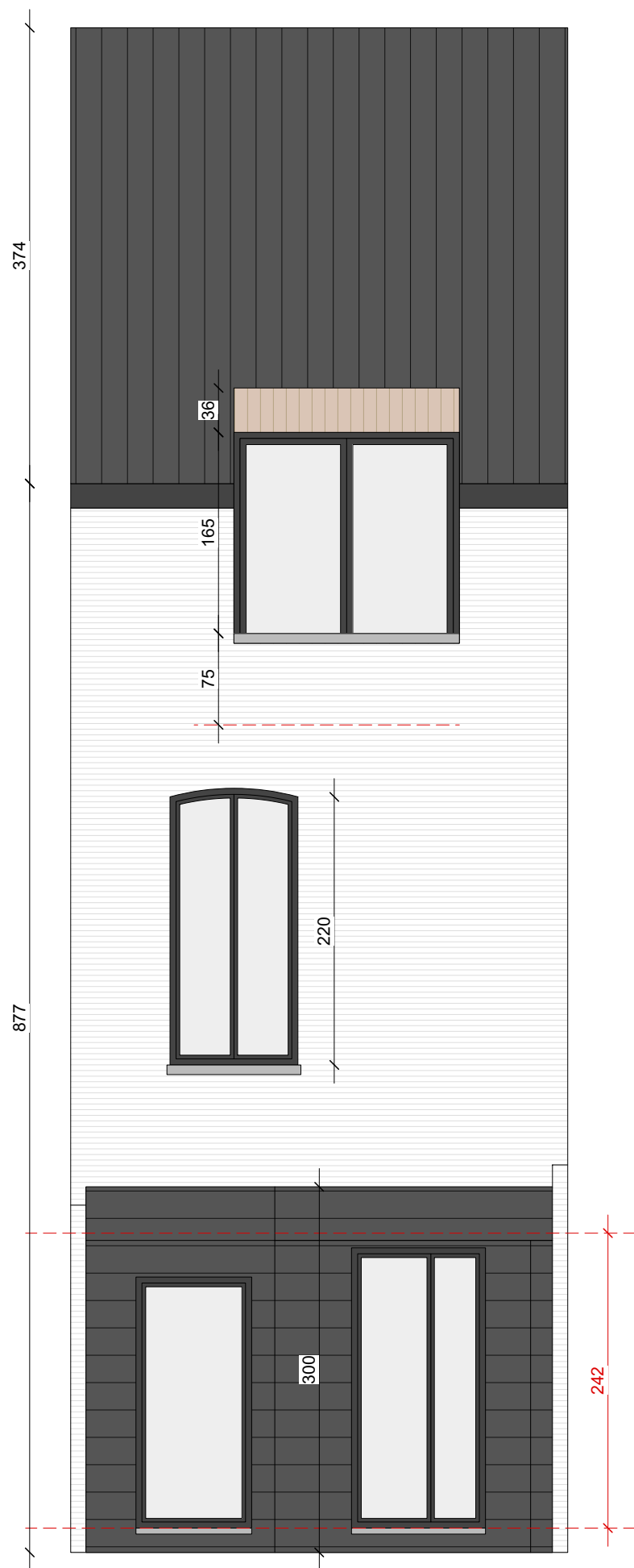
ACHTERGEVEL schaal 1/50
