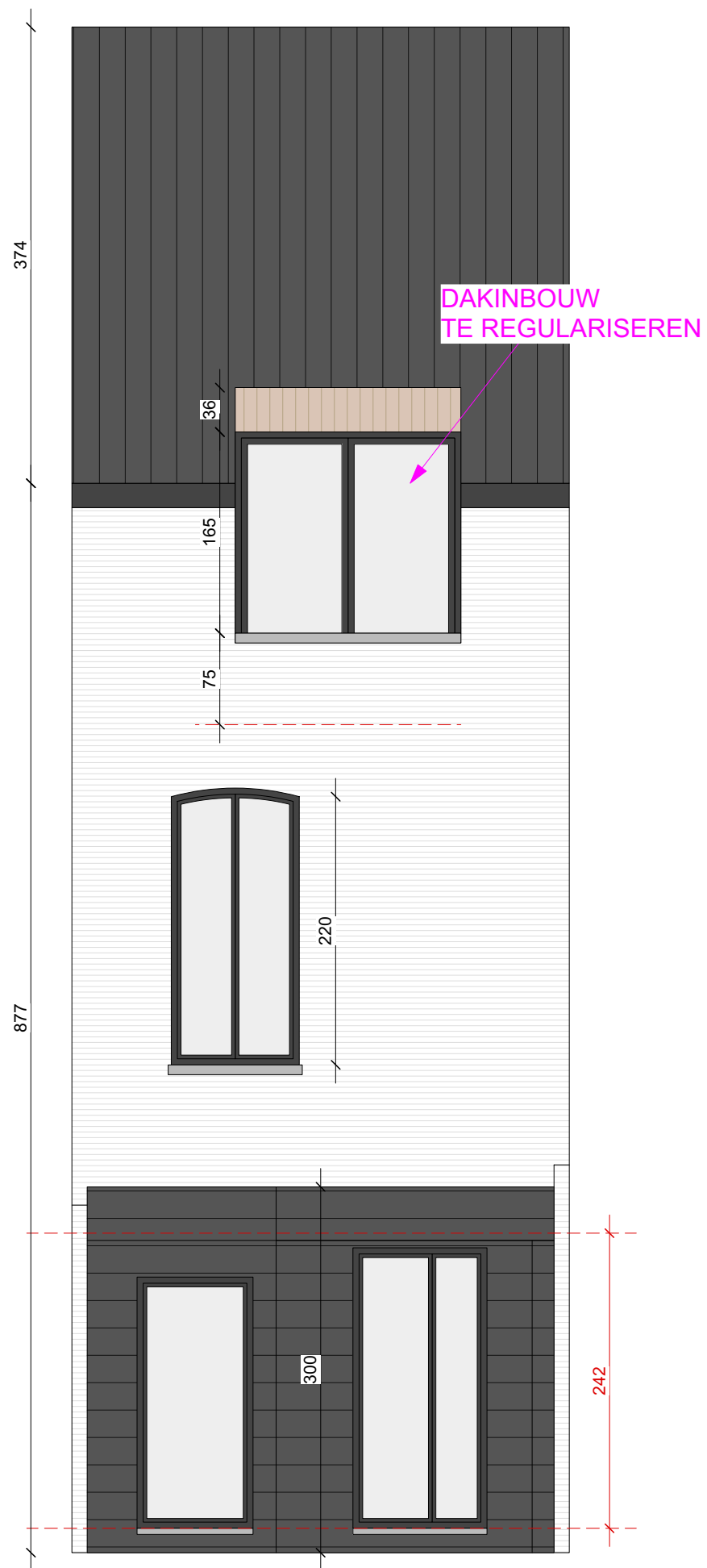
ACHTERGEVEL schaal 1/50
